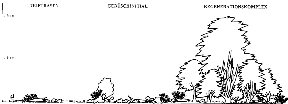
Abb. 2: Schematisierte Entwicklungsreihe einer Hudelandschaft im Villarricagebiet.
