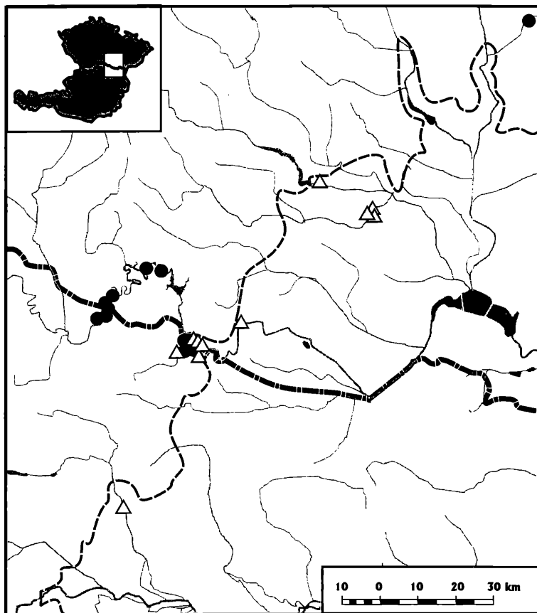
Abb. 1: Verbreitung des Inulo oculi-christi-Stipetum pulcherrimae (△) und des Genisto tinctoriae-Stipetum joannis (●) am Südostrand der Böhmisches Masse mit eingezeichneter Isotherme der 8 °C Jahresmitteltemperatur
