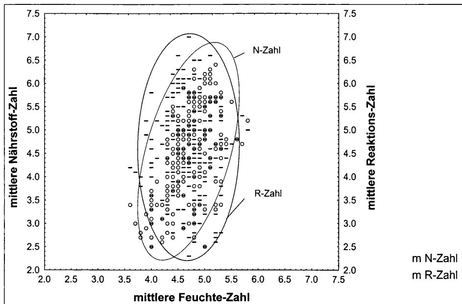
Abb. 2: Ökogramm der Vegetationsaufnahmen mit Cytisus scoparius . Dargestellt sind ungewichtete Zeigerwerte nach ELLENBERG et al. (1992), berechnet aus der Kraut- und Strauchschicht ohne C. scoparius . Die Ellipsen kennzeichnen den jeweiligen 95 %-Konfidenzbereich.
