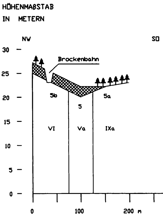
Abb. 8: Sattelmoor zwischen Brocken und Heinrichshöhe. Längsprofil mit Vermoorungsalter (Pollenzonen) (SCHMÜSER 1998 aus BEUG et al. 1999).
