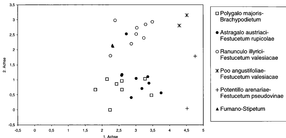
Abb. 2: Ergebnis einer Ordination (DCA) der Aufnahmen.
