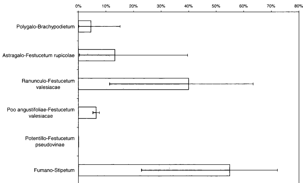
Abb. 3: Anteil der Kies-Fraktion am Gesamtrockengewicht des Bodens. Balken: Mittelwert für die Assoziation, dünne Linie: Variationsbereich.
