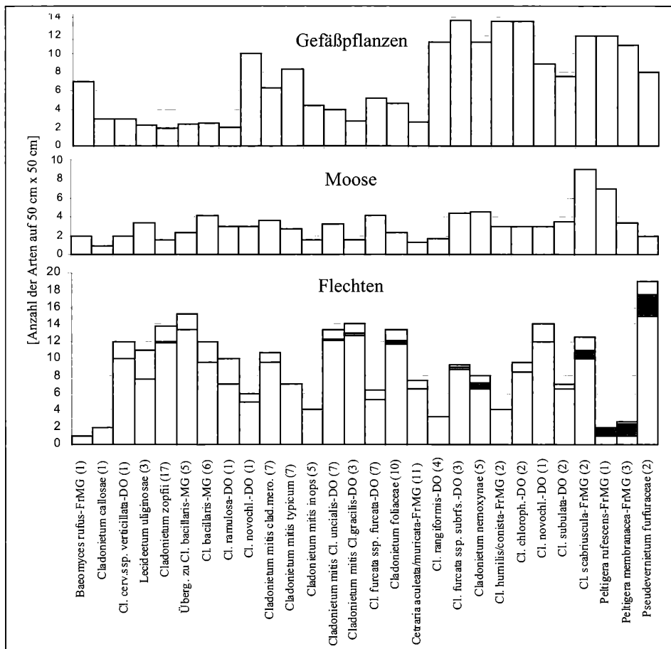
Abb. 3: Anteil am Artenreichtum auf 50 cm x 50 cm großen Aufnahmefflächen: Gefäßpflanzen, Moose und Flechten und Wuchsformen der Flechten (hellgrau: Strauchflechten, dunkelgrau Krustenflechten, schwarz: Blattflechten).
