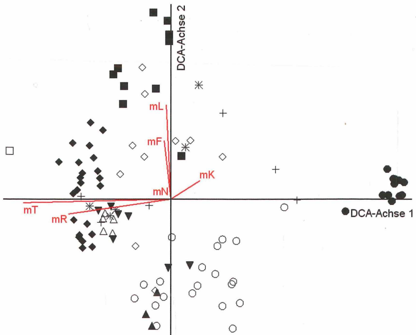
Abb. 7: DCA von Vegetationsaufnahmen mit Lathraea squamaria in Süddeutschland ( n = 102 ) unter Einbeziehung der mittleren, ungewichteten Zeigerwerte für Licht (mL), Temperatur (mT), Kontinentalität (mK), Feuchtigkeit (mF), Bodenreaktion (mR) und Stickstoffversorgung (mN) nach ELLENBERG et al. (2001).
