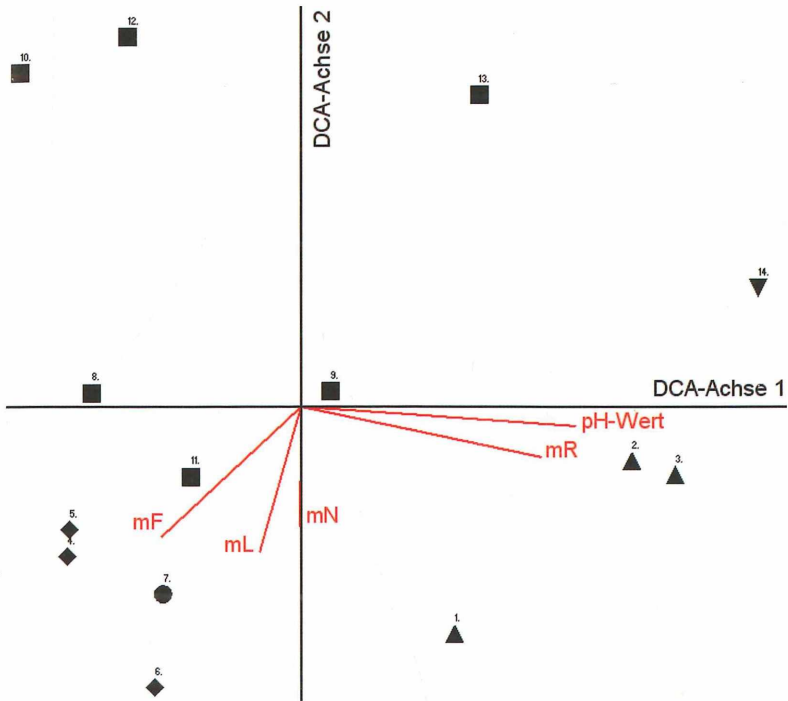
Abb. 3: DCA der Vegetationsaufnahmen mit Lathraea squamaria im Raum Regensburg ( n = 14 ) unter Einbeziehung der mittleren pH( \text{CaCl}_2 )-Werte und der mittleren, ungewichteten Zeigerwerte für Licht (mL), Feuchtigkeit (mF), Bodenreaktion (mR) und Stickstoffversorgung (mN) nach ELLENBERG et al. (2001).
