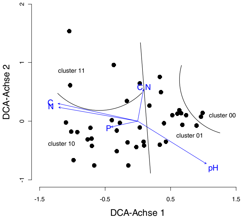
Abb. 4. DCA-Ordinationsdiagramm (Achsen 1 und 2) der 39 Aufnahmen des Wümme-Datensatzes. Die Linien trennen die Datenpunkte der vier TWINSpan-Cluster (s. Tabelle 1) ab. Die Pfeile spiegeln als Post-Hoc -Korrelation die Richtung und Größe des Einflusses der fünf Umweltfaktoren (pH-Wert, Gehalte an pflanzenverfügbarem P, N_{ges} und C_{ges} , C/N-Verhältnis) wider.
