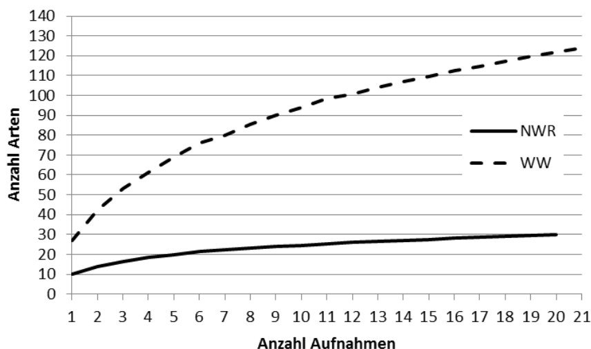
Abb. 5. Arten-Akkumulationskurven für die Aufnahmen aus NWR ( n = 20 ) und WW ( n = 21 ).
