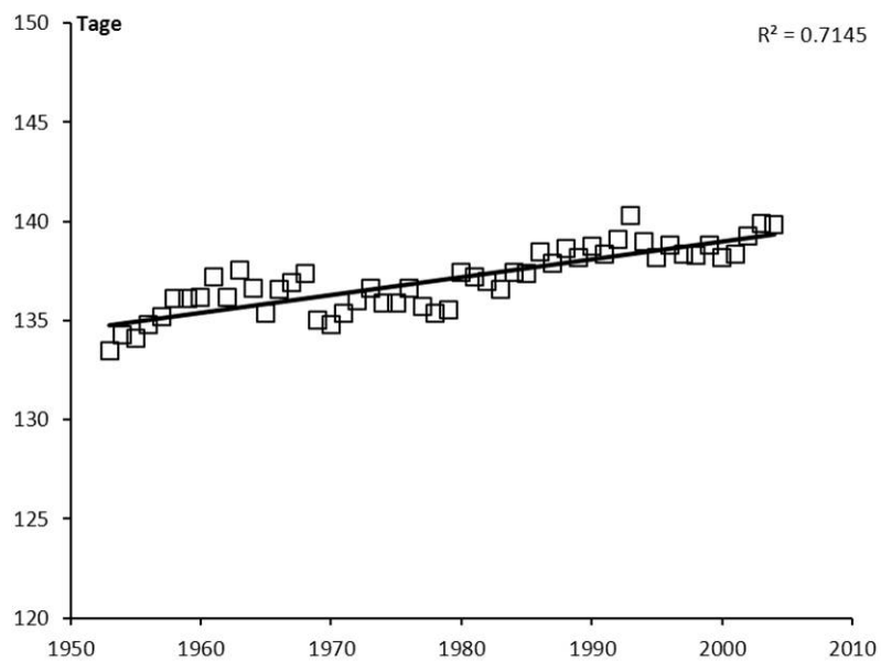
Abb. 2. Gleitendes 10-jähriges Mittel der schneefreien Tage der Vegetationsperiode (01.05.–30.09.) von 1953 bis 2004 mit linearer Trendlinie für Obergurgl (INSTITUTE OF METEOROLOGY AND GEOPHYSICS 2013).
