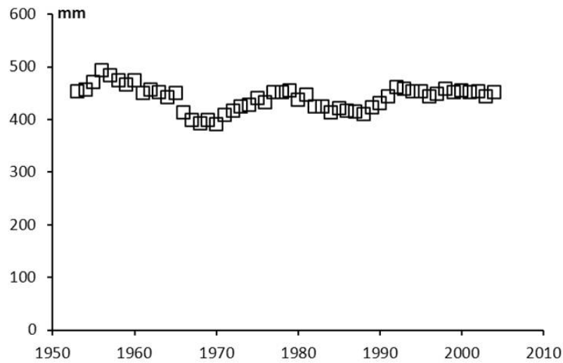
Abb. 1. Gleitendes 10-jähriges Mittel der Sommerniederschläge (Mai – September) von 1953 bis 2004 in Obergurgl (Datengrundlage: INSTITUTE OF METEOROLOGY AND GEOPHYSICS 2013).
