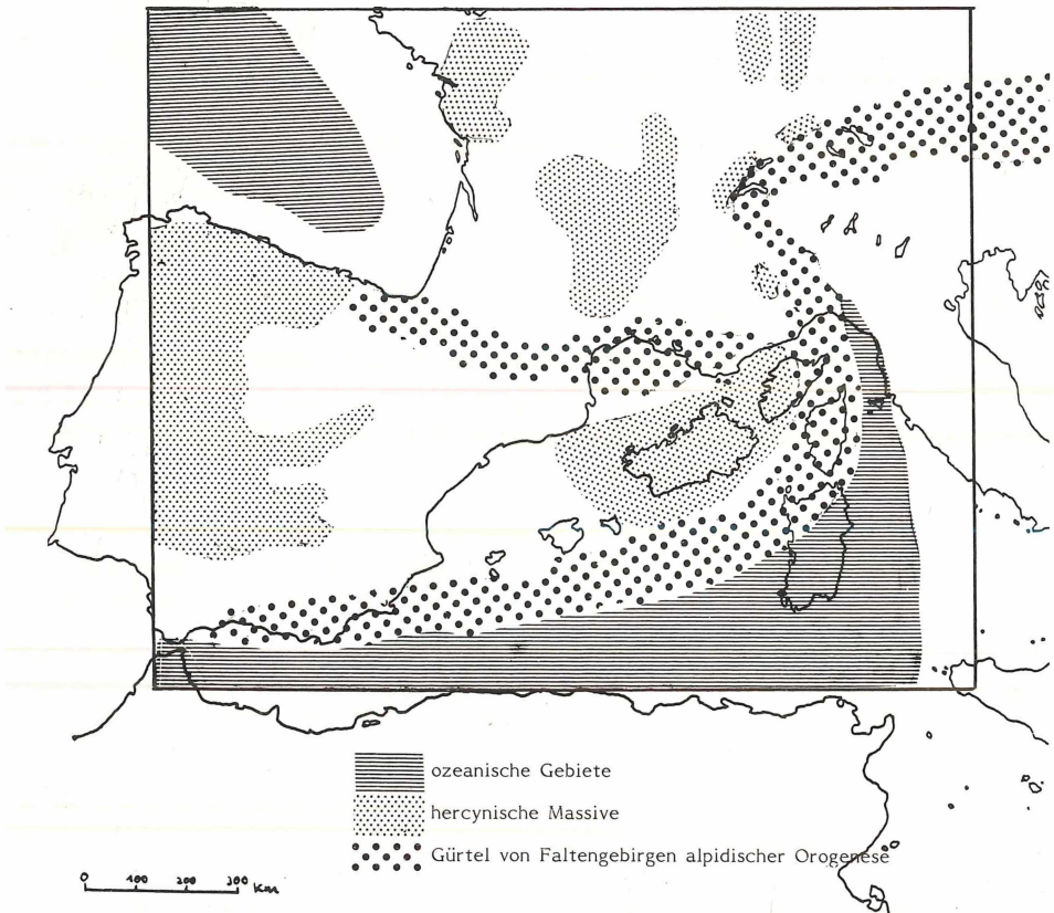
Abb. 3: Rekonstruierte Lage der westmediterranen Landmassen im Oligozän (vor ca. 30 Mio. Jahren) vor Rotation der Korsardischen Platte ("Protoligurisches Massiv"). Die heutige Lage von Korsika und Sardinien ist ebenfalls eingezeichnet. (Nach CARDONA & CONTANDRIOPOULOS, 1979)
