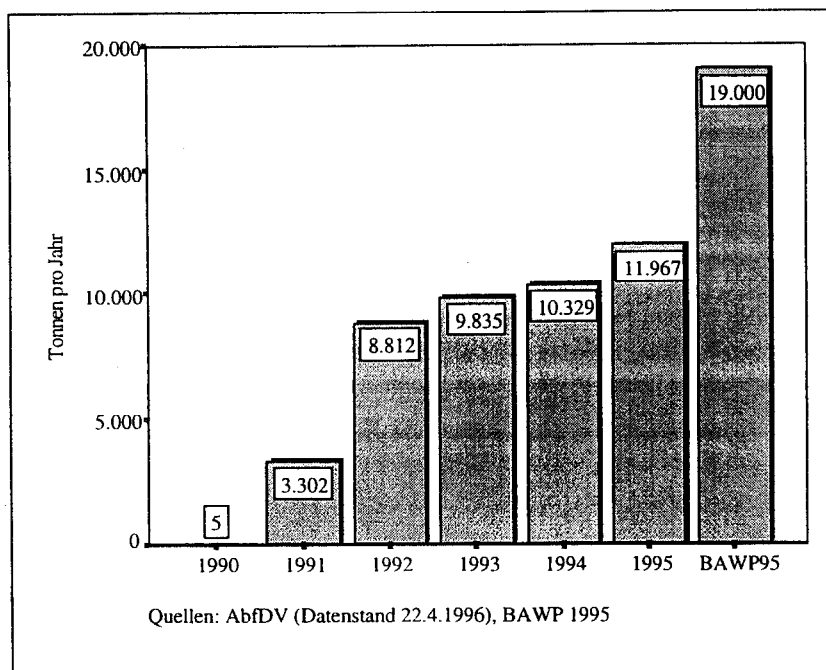
Abbildung 16: Bleiakkumulatoren (SN 35322)
