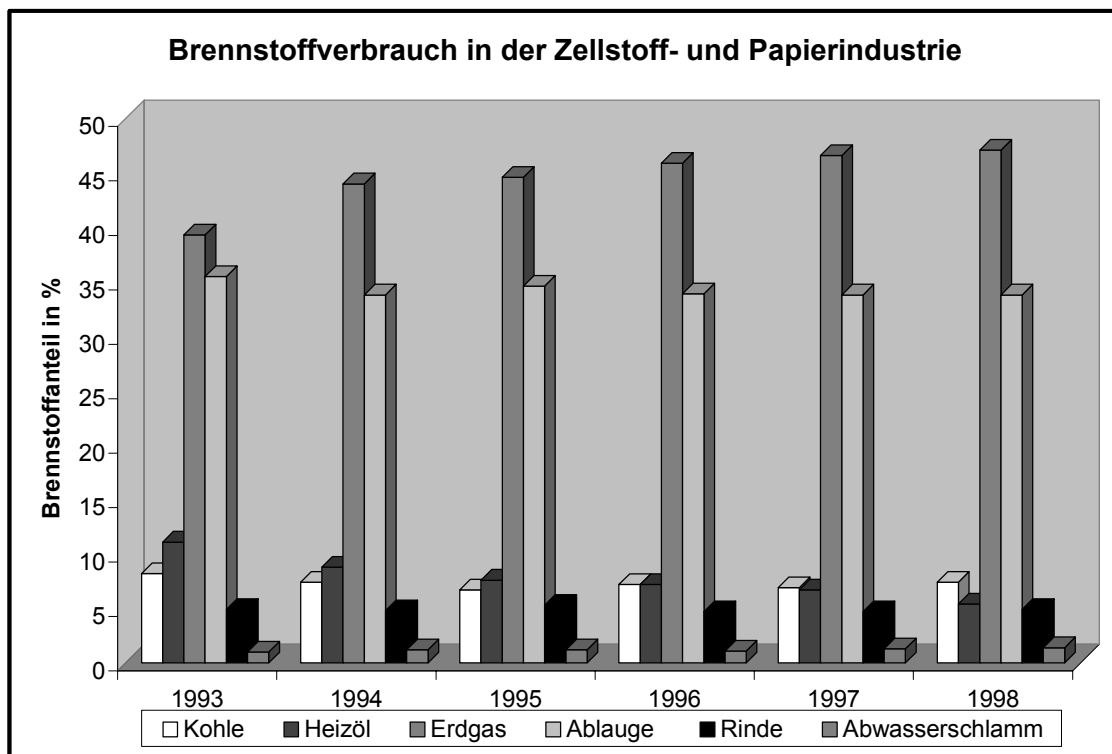
Abb. 3-8: Änderung des Brennstoffverbrauchs in der österreichischen Zellstoff- und Papierindustrie im Lauf der Jahre bezogen auf den Gesamtenergieverbrauch
