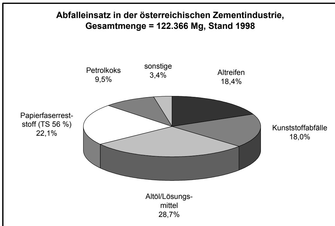
Abb. 3-3: In der österreichischen Zementindustrie im Jahr 1998 eingesetzte Abfallfraktionen
