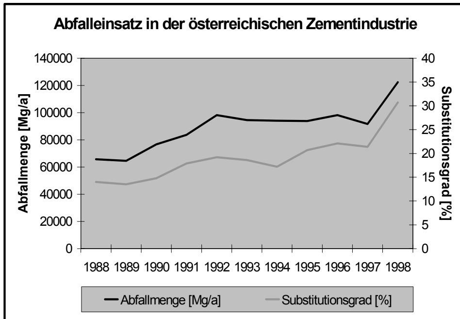
Abb. 3-2: Entwicklung des Abfalleinsatzes und des Substitutionsgrades in der österreichischen Zementindustrie
