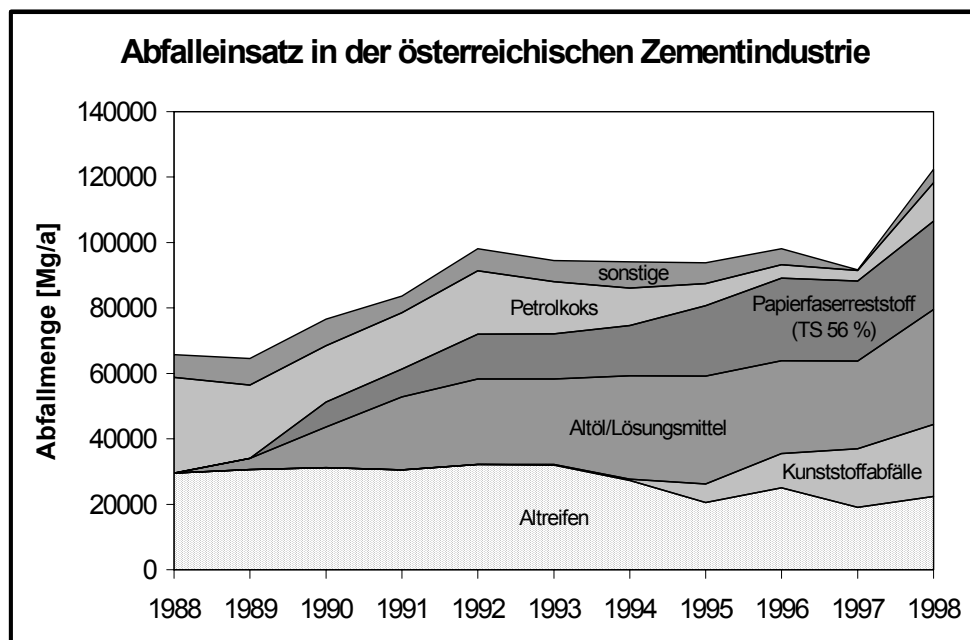
Abb. 3-5: Änderung des Abfalleinsatzes in der österreichischen Zementindustrie im Lauf der Jahre, Darstellung der Gesamtentwicklung
