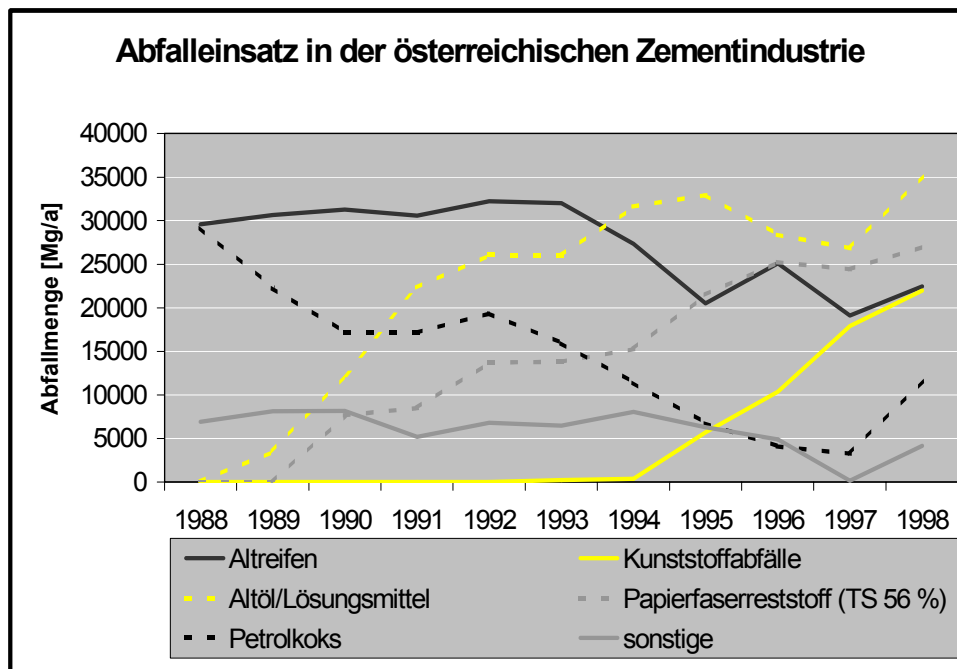
Abb. 3-4: Änderung des Abfalleinsatzes in der österreichischen Zementindustrie im Lauf der Jahre, Darstellung der Entwicklung der einzelnen Fraktionen
