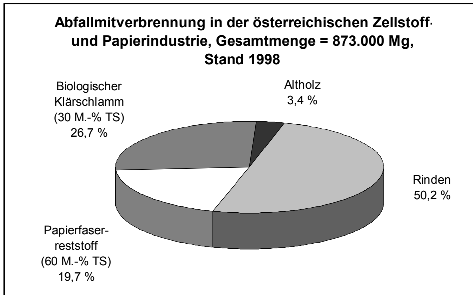
Abb. 3-9: Abfallmitverbrennung in der österreichischen Zellstoff- und Papierindustrie
