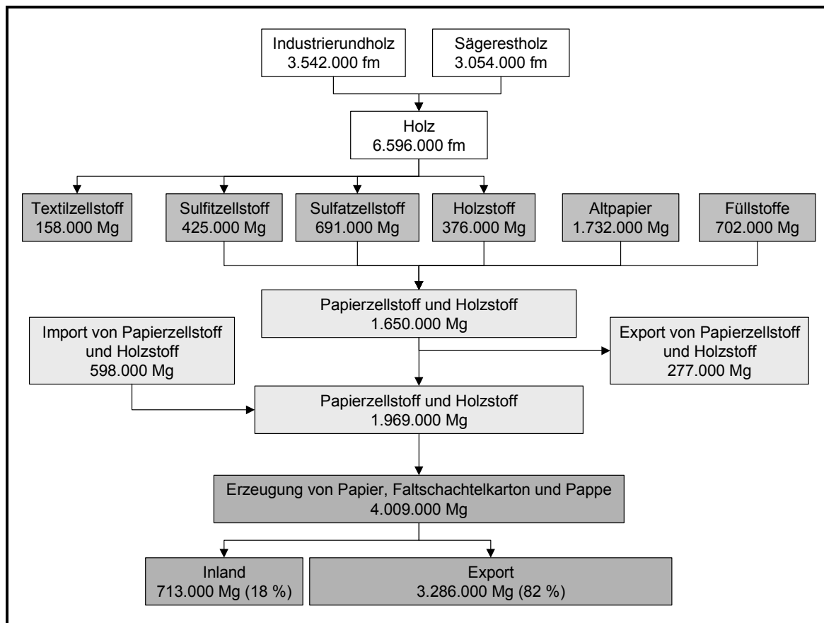
Abb. 3-6: Stoffströme in der österreichischen Zellstoff- und Papierindustrie
