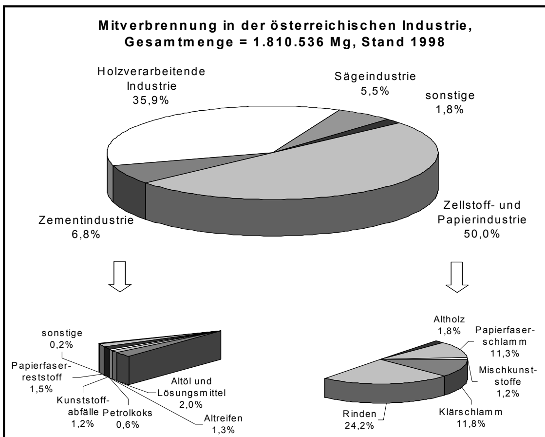
Abb. 4-1: Mitverbrennung in der österreichischen Industrie geordnet nach Branchen, Stand 1998 Bei der Zellstoff- und Papierindustrie sind die Mengen der Reststoffverwertung Lenzing enthalten.
