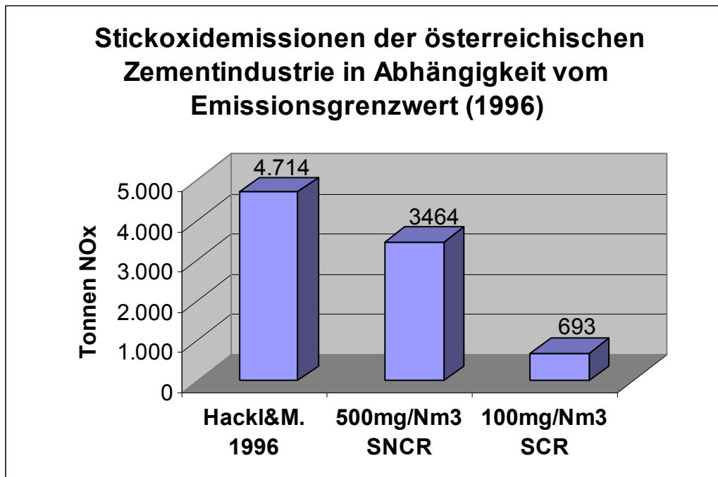
Abbildung 2 \text{NO}_x -Minderungspotential bei der österreichischen Zementindustrie
