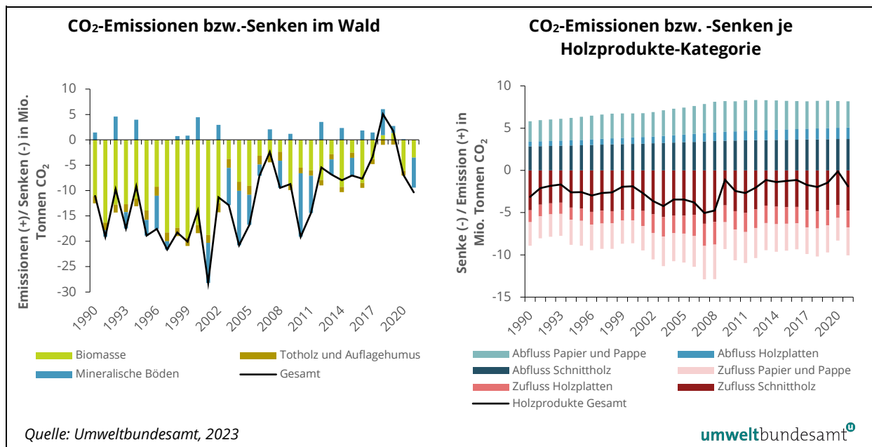
Abbildung 5: Senken und Quellen von Kohlendioxid im österreichischen Wald und in Holzprodukten von 1990 bis 2021.
