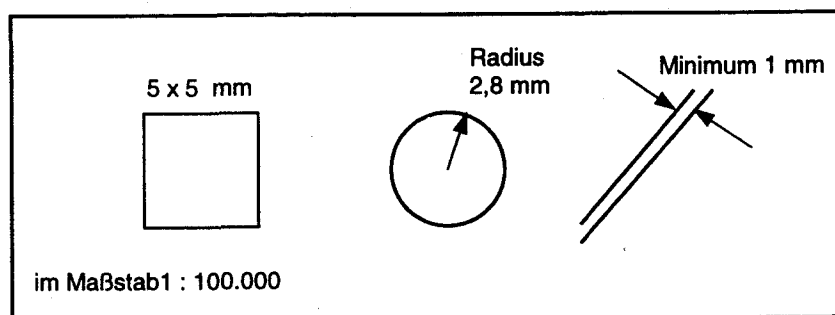
Abb. 4: Kleinste Erhebungseinheiten
