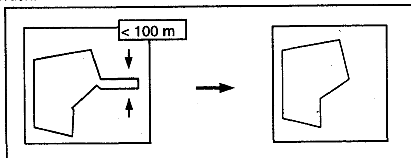
Abb. 10: Vereinfachungen, Glätten
