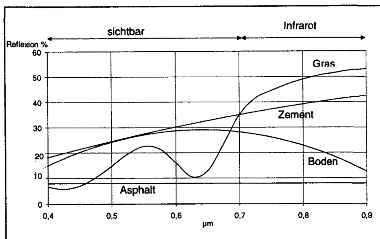
Abb. 2: Boden, Reflexionsvermögen
