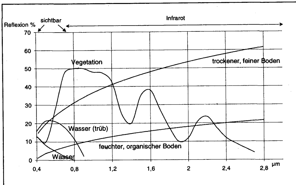
Abb. 1: Reflexionsvermögen von Vegetation 1
