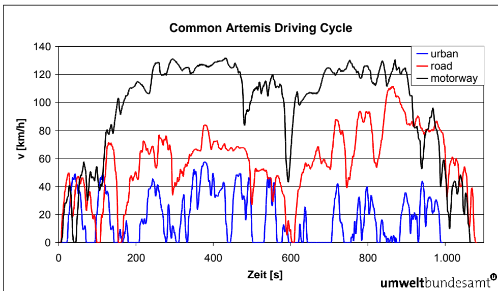
Abbildung 2: Geschwindigkeitsverlauf CADC (Common Artemis Driving Cycle).
