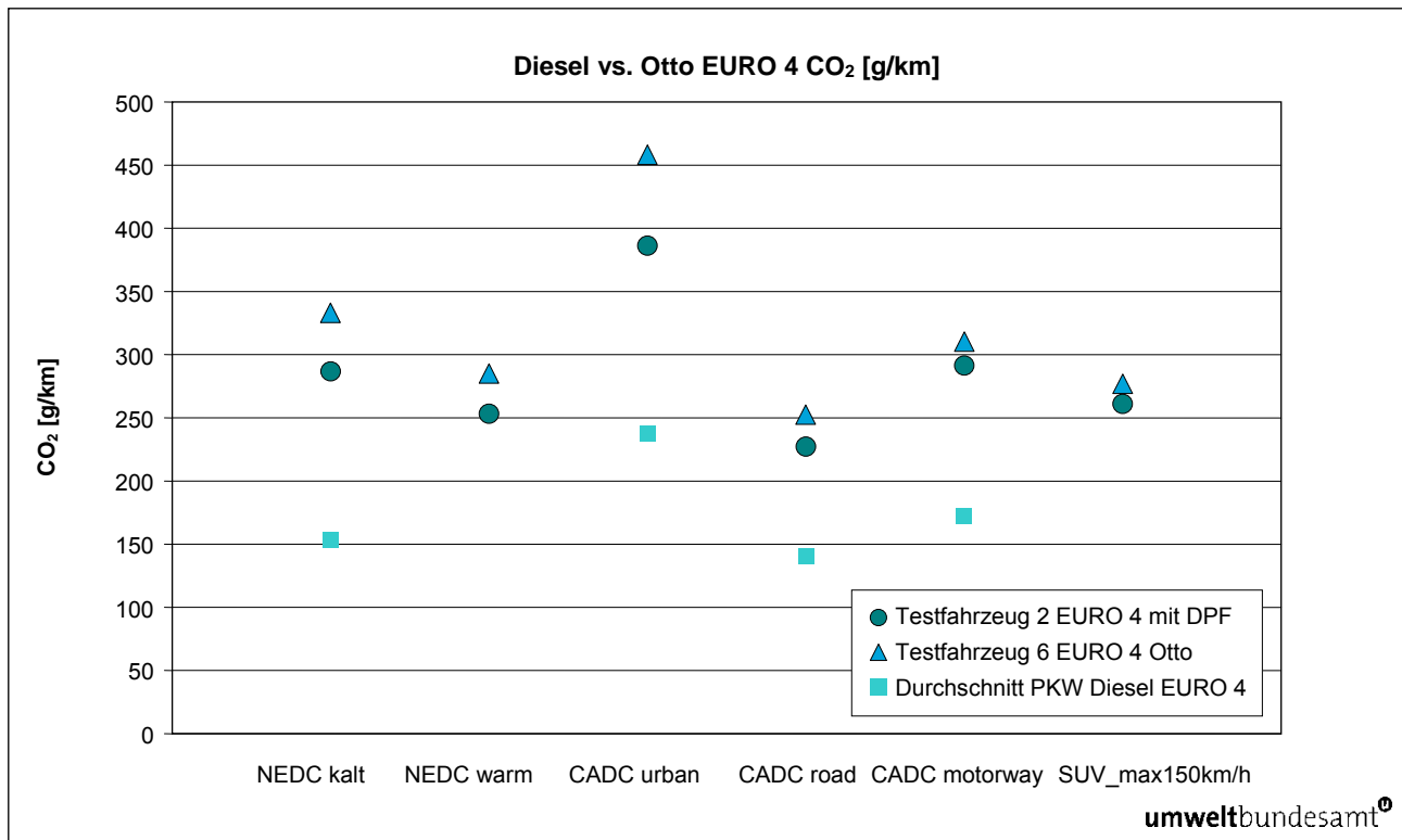
Abbildung 14: CO 2 – Vergleich zwischen Diesel- und Otto-Fahrzeug.
