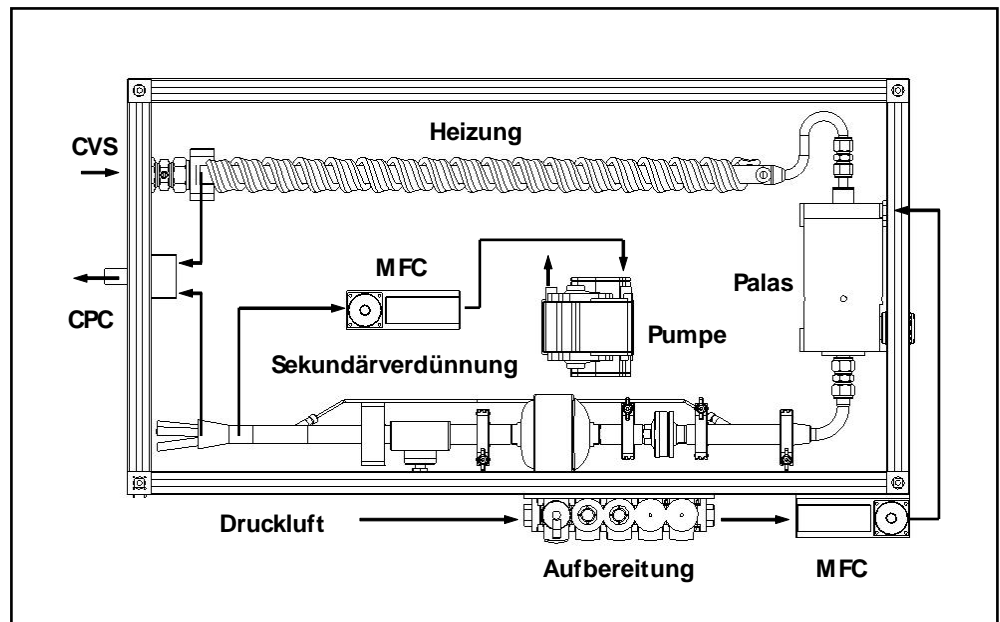
Abbildung 4: System zur Probennahme bei der Partikelanzahlmessung (SCHMÖLZER 2006).
