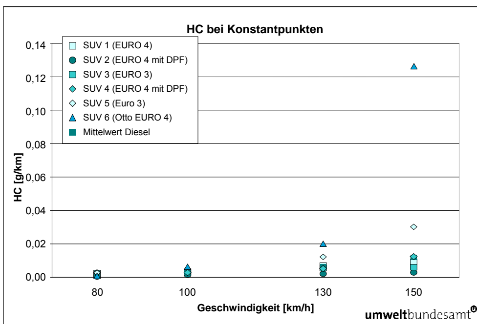
Abbildung 24: HC-Emissionen bei konstanten Geschwindigkeiten.
