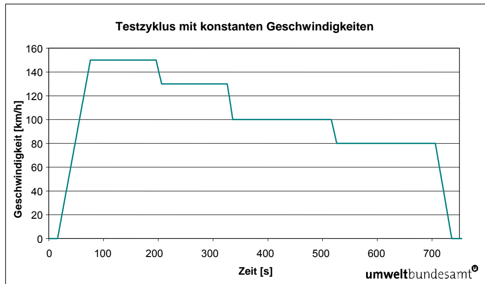
Abbildung 3: Geschwindigkeitsverlauf des Testzyklus „SUV_max150km/h“ mit konstanten Geschwindigkeiten.
