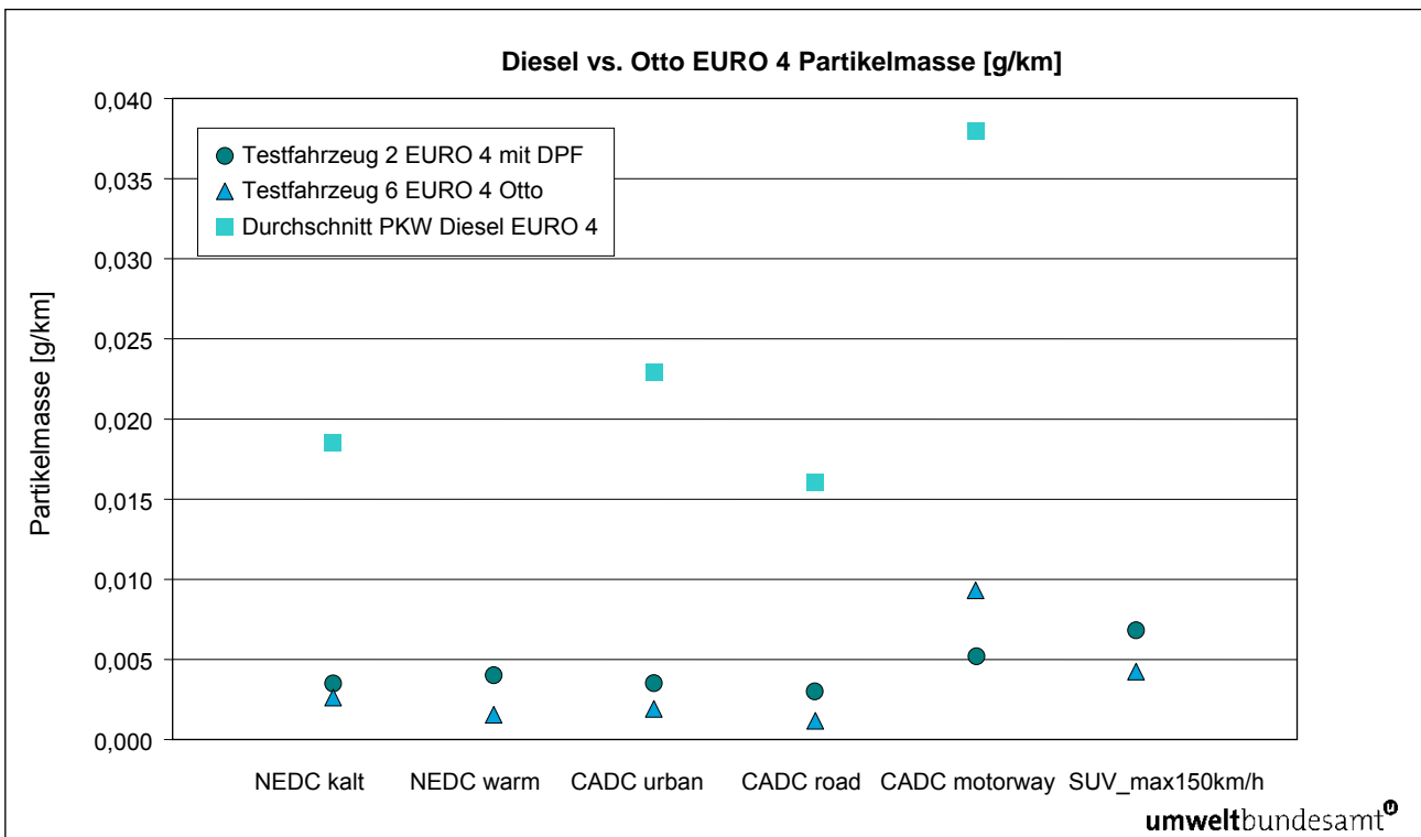
Abbildung 16: Partikelmasse – Vergleich zwischen Diesel- und Otto-Fahrzeug.
