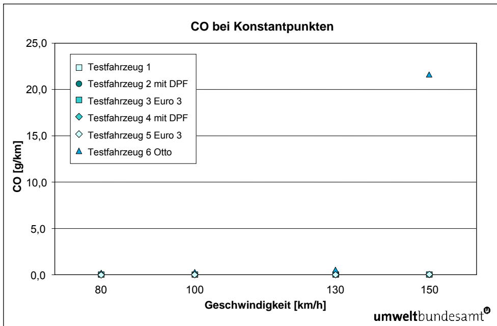
Abbildung 23: CO-Emissionen bei konstanten Geschwindigkeiten.
