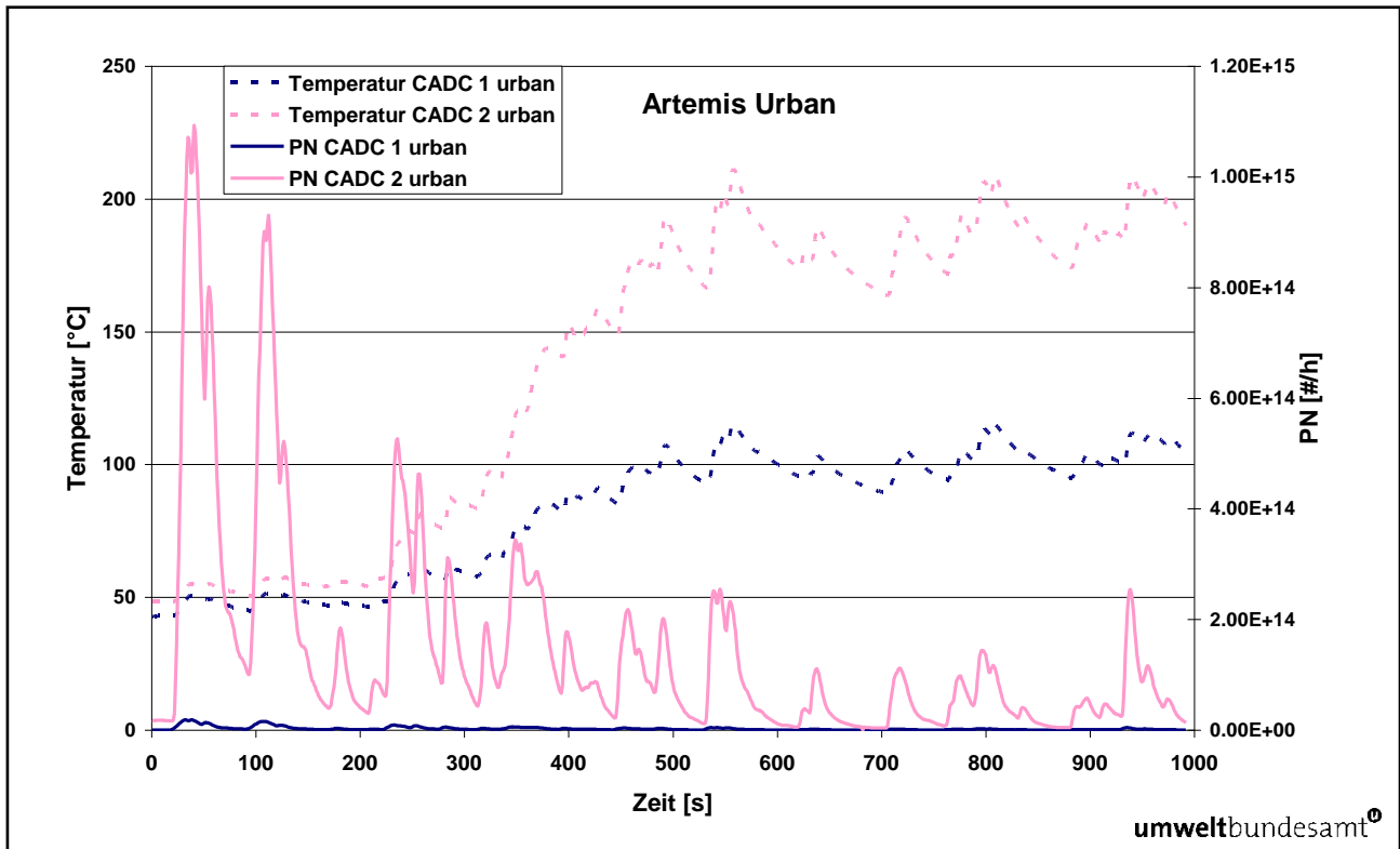
Abbildung 19: Partikelanzahl und Temperaturverlauf (nach Endschalldämpfer) im CADC urban.
