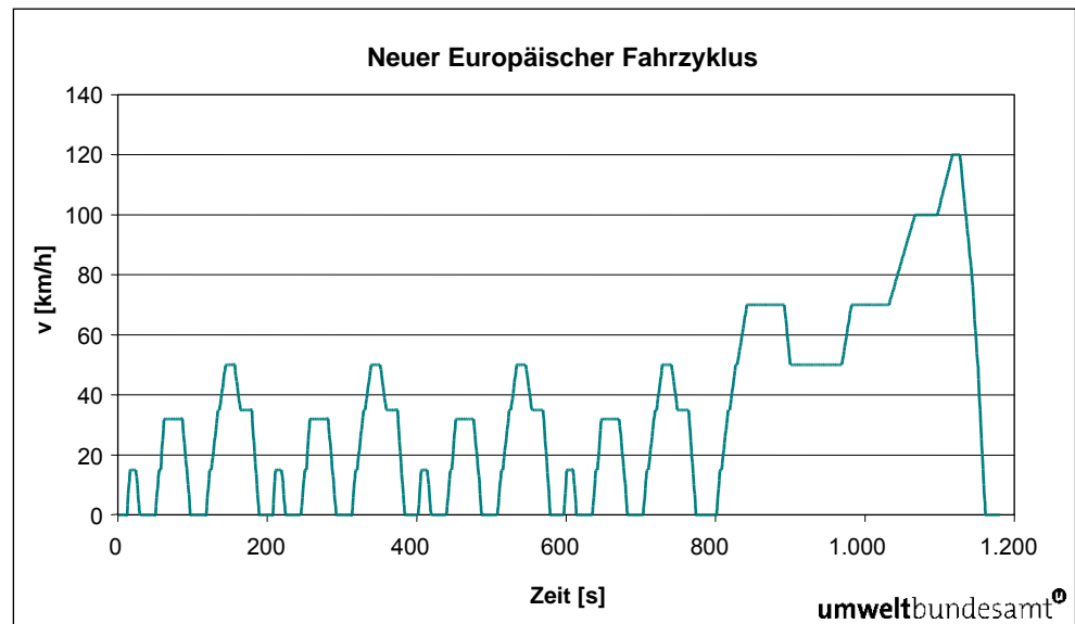
Abbildung 1: Geschwindigkeitsverlauf NEDC (New European Driving Cycle, Neuer Europäischer Fahrzyklus).
