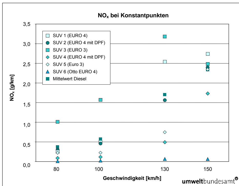
Abbildung 21: NO x -Emissionen bei konstanten Geschwindigkeiten.
