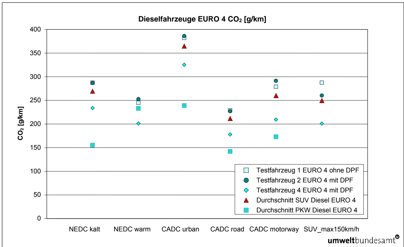
Abbildung 5: CO 2 -Emissionen für EURO 4 Dieselfahrzeuge in den verschiedenen Testzyklen.
