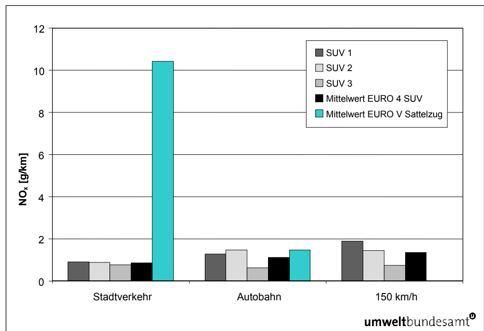
Abbildung 22: \text{NO}_x -Emissionen von EURO 4 SUV und EURO 5 Sattelzügen im Vergleich.
