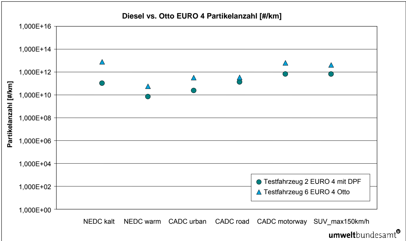
Abbildung 17: Partikelanzahl – Vergleich zwischen Diesel- und Otto-Fahrzeug.
