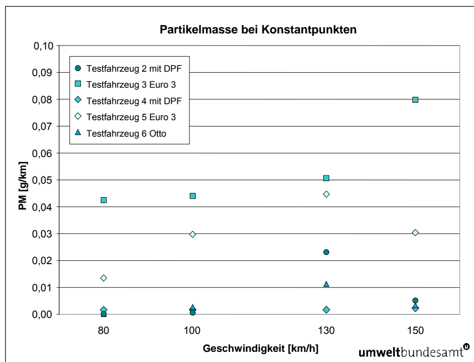
Abbildung 26: Partikelmasse bei konstanter Geschwindigkeit.
