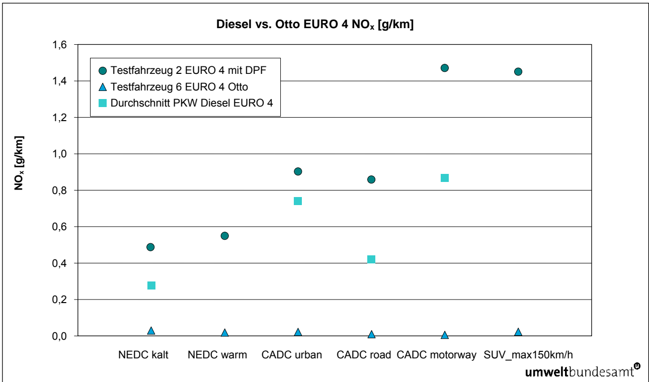
Abbildung 15: NO x – Vergleich zwischen Diesel- und Otto-Fahrzeug.
