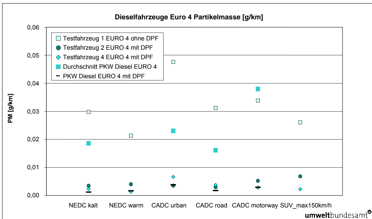
Abbildung 9: Partikelmasse für EURO 4 Dieselfahrzeuge in den verschiedenen Testzyklen.
