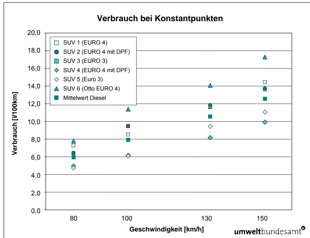
Abbildung 20: Verbrauch der 6 Testfahrzeuge bei konstanten Geschwindigkeiten.
