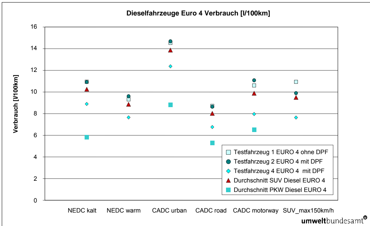
Abbildung 6: Verbrauch [l/km] für EURO 4 Dieselfahrzeuge in den verschiedenen Testzyklen.
