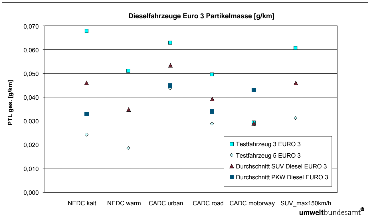
Abbildung 13: Partikelmasse für EURO 3 Dieselfahrzeuge in den verschiedenen Testzyklen.
