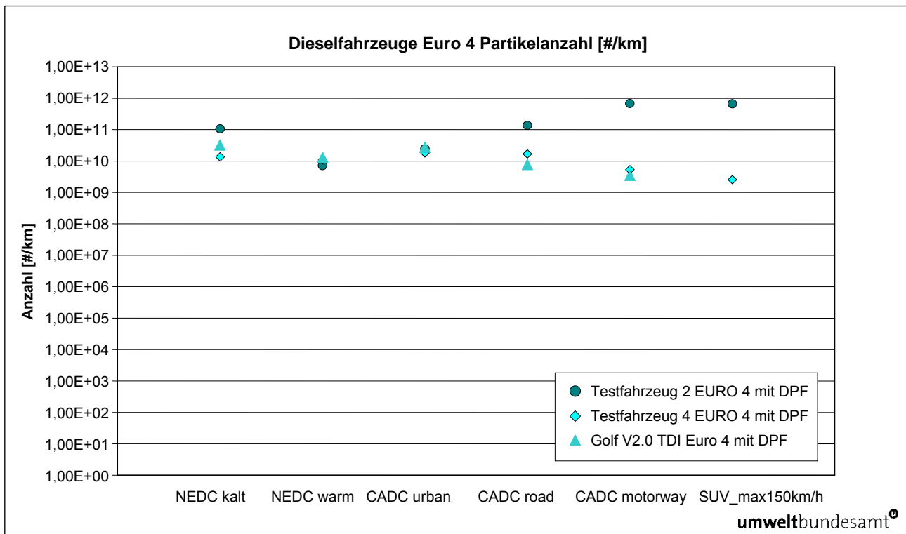
Abbildung 10: Partikelanzahl für EURO 4 Dieselfahrzeuge in den verschiedenen Testzyklen.
