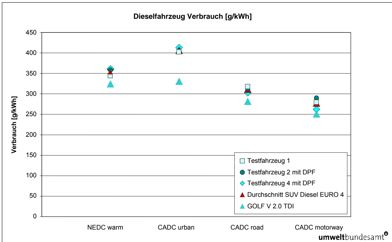
Abbildung 7: Verbrauch [g/kWh] für EURO 4 Dieselfahrzeuge in den verschiedenen Testzyklen.
