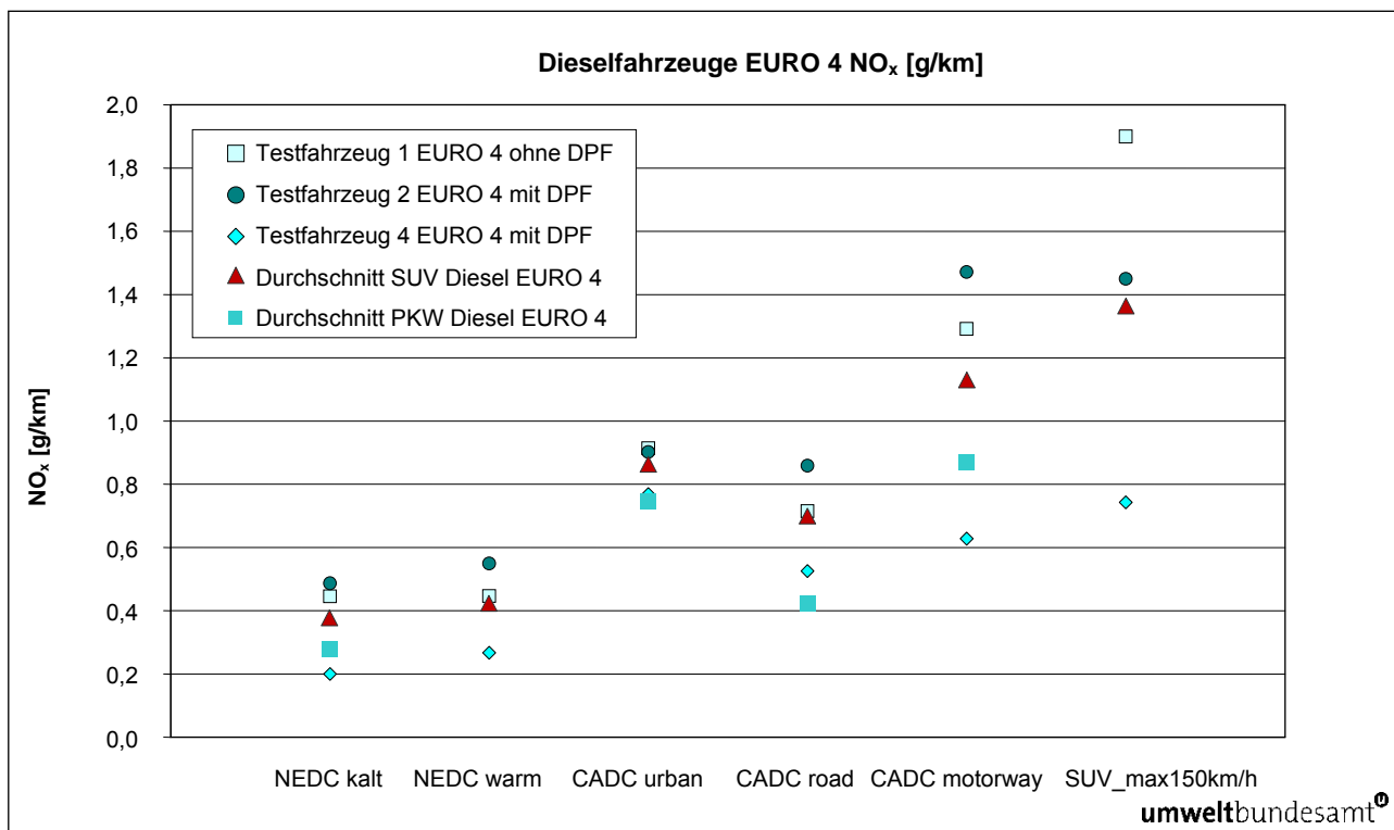
Abbildung 8: NO x -Emissionen für EURO 4 Dieselfahrzeuge in den verschiedenen Testzyklen.
