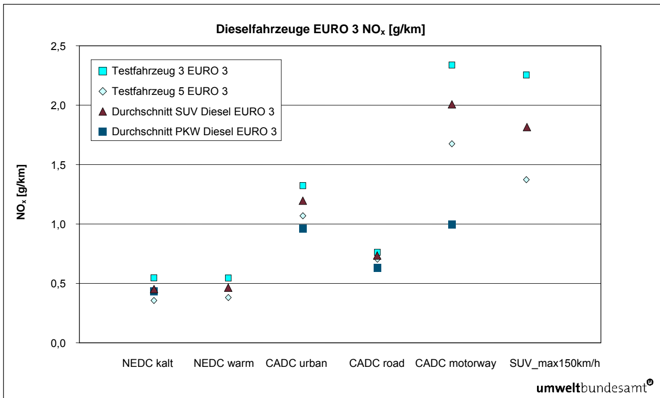
Abbildung 12: NO x -Emissionen für EURO 3 Dieselfahrzeuge in den verschiedenen Testzyklen.
