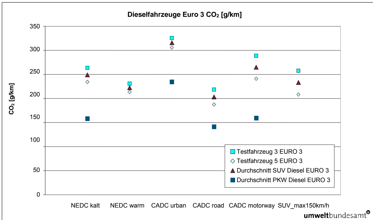
Abbildung 11: CO 2 -Emissionen für EURO 3 Dieselfahrzeuge in den verschiedenen Testzyklen.
