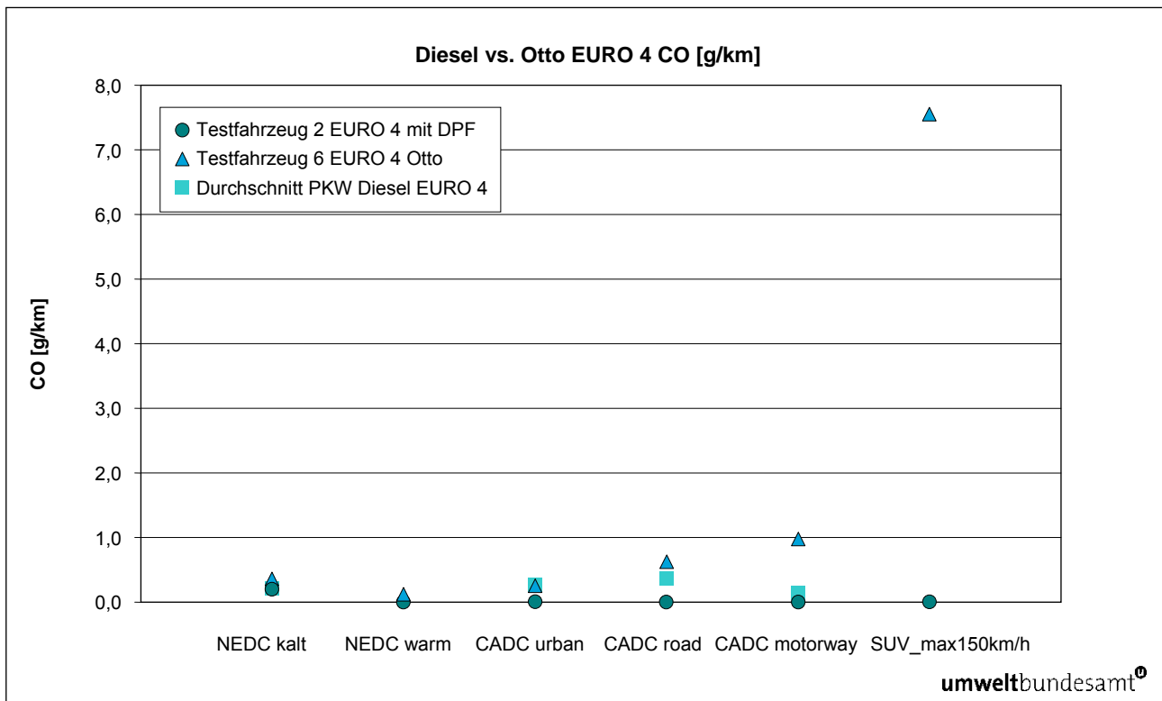
Abbildung 18: CO – Vergleich zwischen Diesel- und Otto-Fahrzeug.
