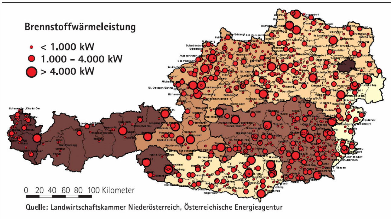
Abbildung 12: Verteilung der Biomasseheiz- und -Heizkraftwerke in Österreich 2005 (EA et al. 2006).
