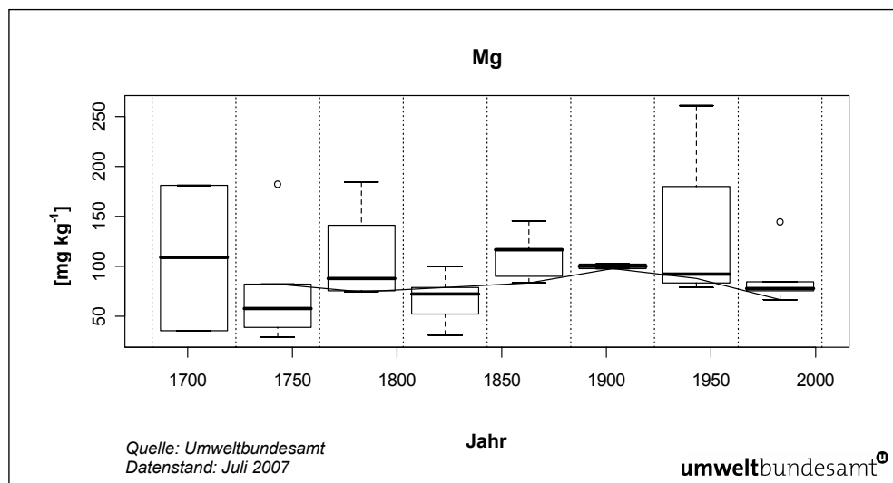
Abbildung 21: Historische Entwicklung des Magnesiumgehaltes (mg kg -1 ).
