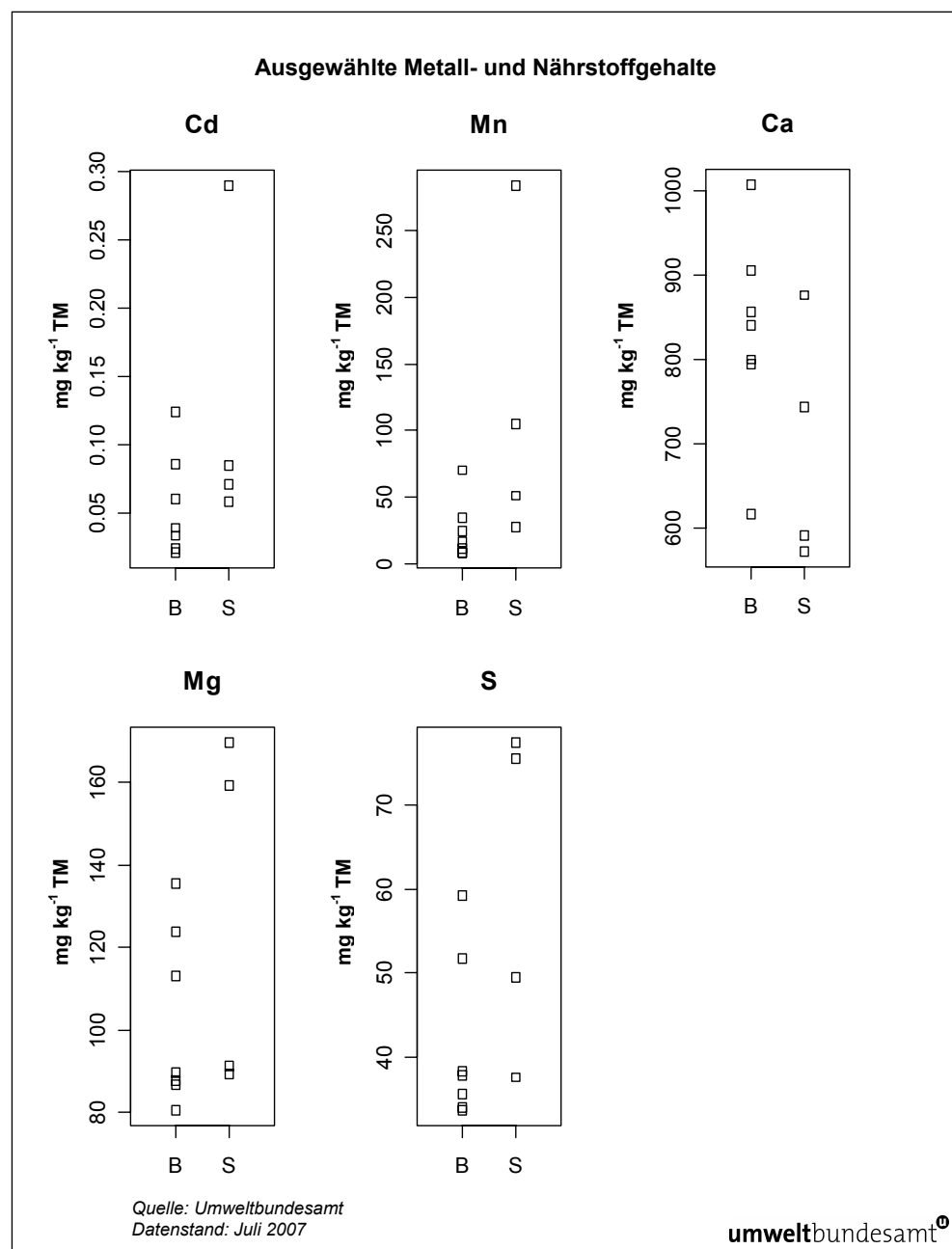
Abbildung 5: Ausgewählte Metall- und Nährstoffgehalte ( \text{mg kg}^{-1} lufttrocken) auf Standorten mit unterschiedlicher Bodenreaktion (B ... basisch, S ... sauer).
