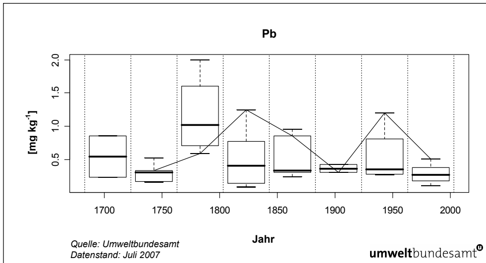
Abbildung 9: Historische Entwicklung des Bleigehaltes ( \text{mg kg}^{-1} ).
