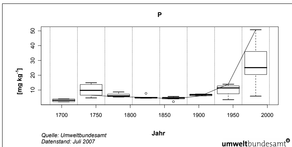
Abbildung 24: Historische Entwicklung des Phosphorgehaltes ( \text{mg kg}^{-1} ).
