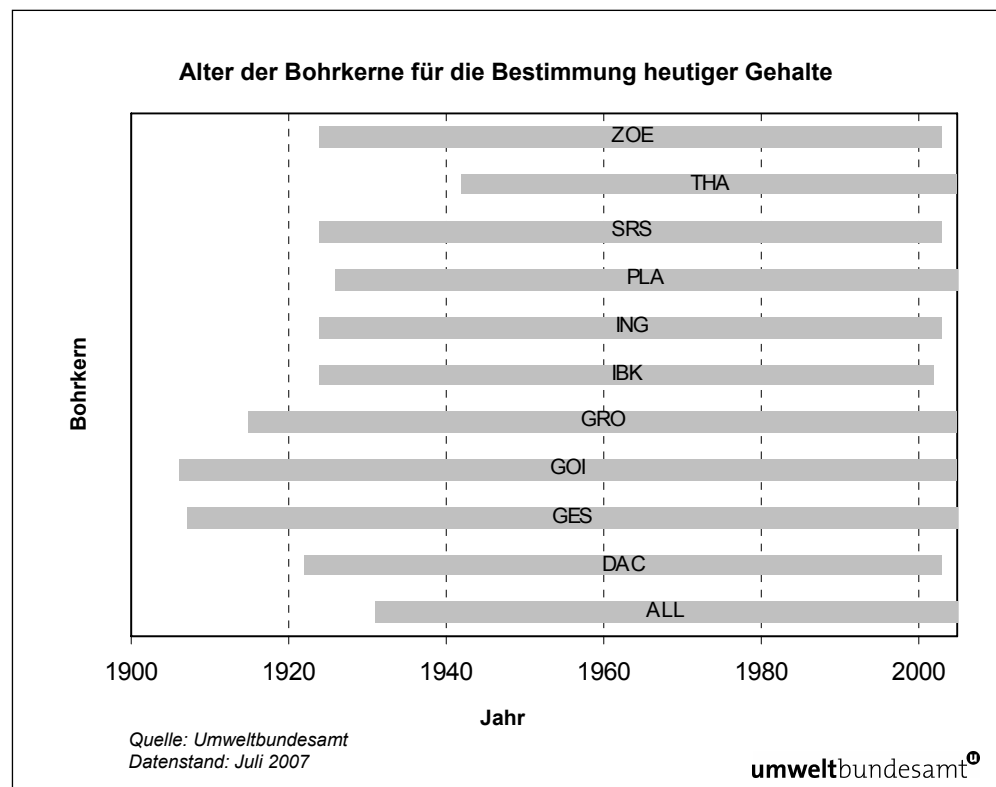
Abbildung 2: Alter der Bohrkerne für die Bestimmung heutiger Gehalte.
