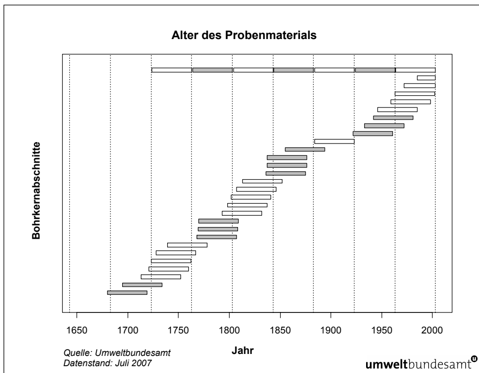
Abbildung 3: Alter des Probenmaterials für die Untersuchung der historischen Entwicklung. Der oberste Balken stellt einen durchgehenden Bohrkern dar, die restlichen Balken symbolisieren Bohrkerneabschnitte verschiedener Individuen. Vertikale punktierte Linien trennen die einzelnen 40-Jahr-Episoden.
