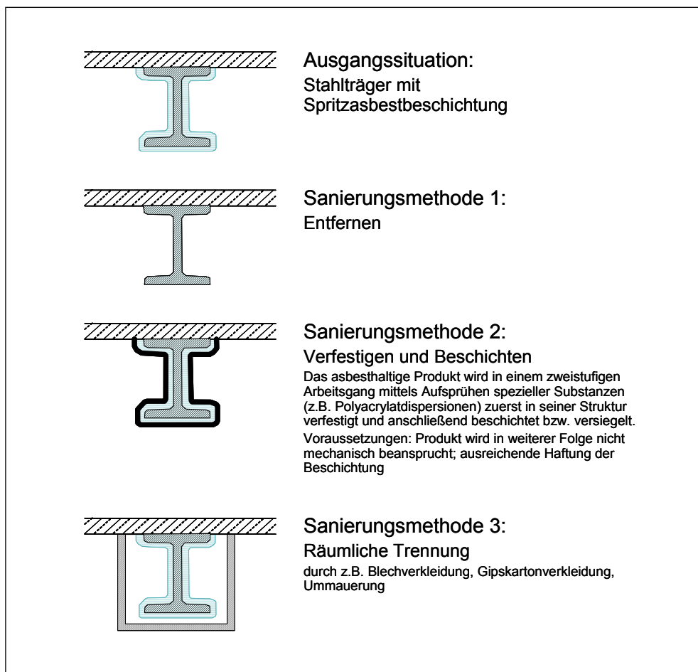
Abbildung 5: Methoden der Asbestsanierung (DWORAK 2002).
