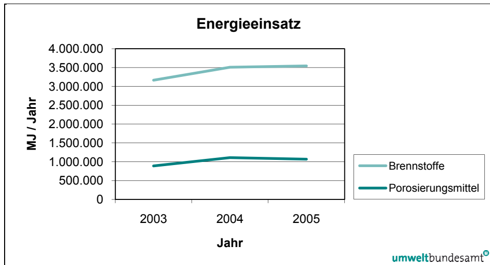
Abbildung 1: Energieeinsatz aus Brennstoffen und Porosierungsmitteln für die Jahre 2003 bis 2005.
