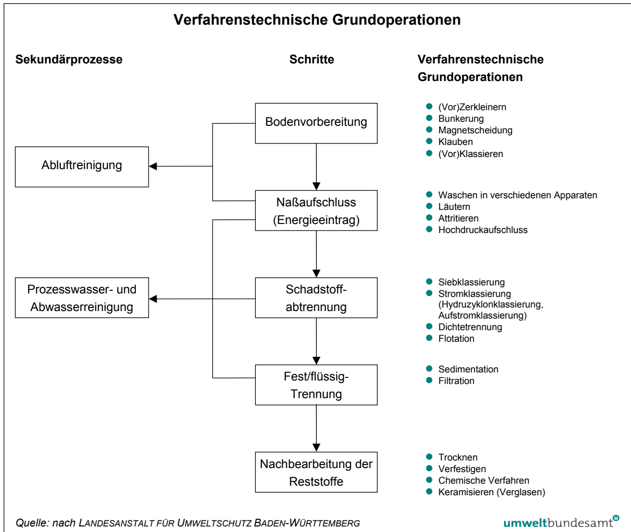
Abbildung 1: Verfahrenstechnische Grundoperationen.
