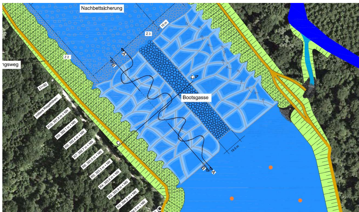
Abbildung 22: Sohlabstufung Fkm 51.9
