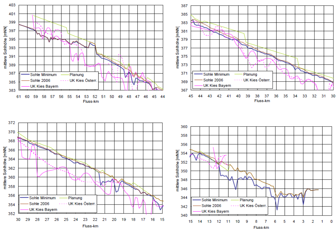
Abbildung 21: Variante B kurz – Vergleich tiefstes Sohlniveau aus der Rechnung mit Planungssohle, geschätzte Sohle 2006 und Unterkante Kieshorizont
