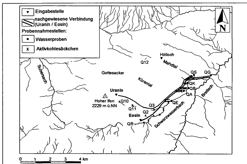
Abb. 18: Gewässernetz und Quellen im Untersuchungsgebiet, Lage der Eingabe- und Probenabnahmestellen während des kombinierten Markierungsversuches und nachgewiesene Verbindungen. Die Verbindung Hölloch-Sägebachquelle (Q5) wurde bereits 1949 und 1955 nachgewiesen
