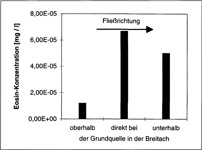
Abb. 22: Eosin-Konzentration in der Breitach am 29.09.1996, oberhalb, direkt bei und unterhalb der Grundquelle (QG) in der Breitach. Die Eosin-Konzentration ist unterhalb der Grundquelle deutlich höher als oberhalb und direkt bei der Grundquelle am höchsten. Dies beweist, daß hier Karstwasser aus dem Gebiet Gottesacker-Schwarzwassertal austritt. Die Grundquelle ist demnach der tiefste Austritt des Karstsystems
