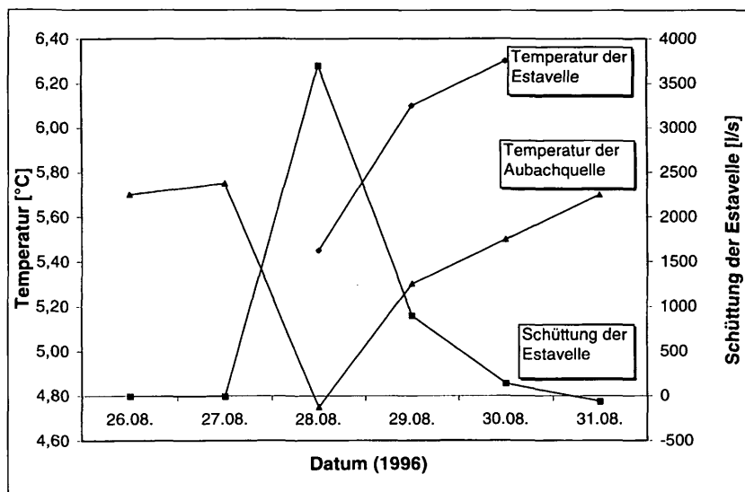
Abb. 10: Zusammenhang zwischen Schüttung und Temperatur der Estavelle und Temperatur der Aubachquelle. Nach starken Niederschlägen fördern Estavelle und Aubachquelle kaltes „Plateauwasser“, das aus dem Gottesacker zuströmt. Bei nachlassender Schüttung der Estavelle steigen die Temperaturen der Aubachquelle, da zunehmend warmes „Talwasser“ gefördert wird
