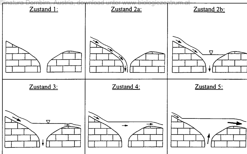
Abb. 9: Beobachtete Zustände der Estavelle: 1) trocken, 2) vollständige Versinkung, a) ohne Pool, b) mit Pool, 3) teilweise Versinkung, 4) neutral, 5) Grundquelle
