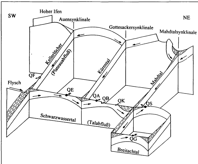
Abb. 25: Hydrogeologische Modellvorstellung des Untersuchungsgebietes (die Pfeile zeigen die Fließbewegung im Karstgrundwasserleiter): Die Synklinalen stellen bevorzugte Entwässerungsbahnen für die vom Gottesacker abfließenden Karstwässer dar (Plateauabfluß). Der im Schwarzwassertal unter den Flysch abtauchende Karstkörper sammelt diese Karstwässer (Talabfluß) und leitet sie an die Karstquellen (QA, QB, QK) weiter. Bei hohen Niederschlägen wird auch die Estavalle (QE) zur Quelle, nach extrem starken Niederschlägen sogar das Fuchslotz (QF). Der Schwarzwasserbach selbst wird aus dem oberen Schwarzwassertal und von oberirdischen Zuflüssen aus dem Flyschgebiet gespeist. Das Grundwasser aus dem Schwarzwassertal fließt unter dem Mahdtal hindurch, um in der Sägebachquelle (QS) wieder zutagezutreten. Im unteren Schwarzwassertal und an der Breitach ist der Schrättkalk von Leismergeln überlagert. Dort, wo der Karstgrundwasserleiter von der Breitach angeschnitten wird, befindet sich die Grundquelle QG, die den tiefsten Auslaß des Karstsystems darstellt
