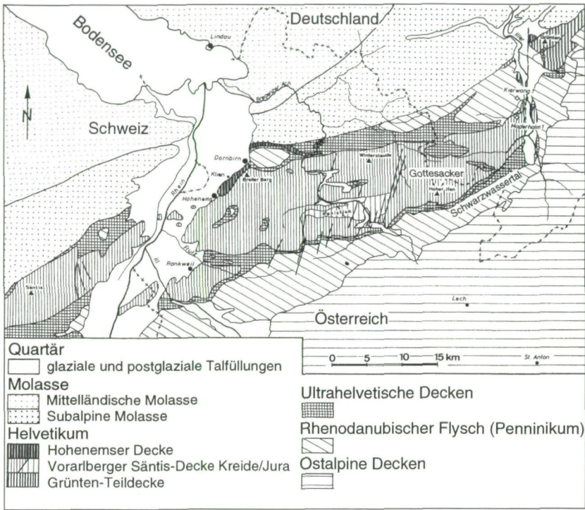
Abb. 2: Geologisch-tektonische Übersichtskarte der Allgäuer und Vorarlberger Alpen. Molasse, Flysch, Helvetikum und Ostalpin sind hier auf engstem Raum nebeneinander anzutreffen. Das Helvetikum bildet ein großes tektonisches Halb-fenster inmitten der Flyschdecken, die es im Norden, Osten und Süden umgeben. Der Gottesacker liegt am Ostrand dieses Halb-fensters, entlang des Schwarzwassertaes taucht das Helvetikum unter die Flyschzone ab (WYSSLING, 1986)
