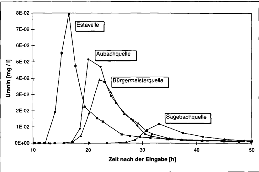
Abb. 21: Uranin-Durchgangskurven aller Probenahmestellen im Vergleich. Je weiter die Entfernung zur Eingabestelle, umso später kommt der Tracer an und umso höher ist die Dispersion
