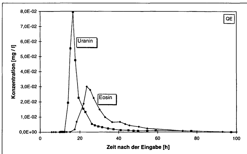
Abb. 20: Tracer-Durchgangskurven der Estavelle, im Schwarzwasserbach unterhalb der Estavelle gemessen
