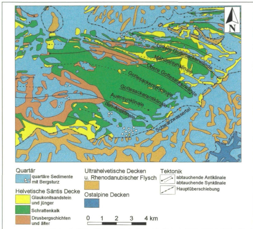
Abb. 4: Vereinfachte Geologische Karte des Gottessackgebietes mit der Lage der abtauchenden Faltenachsen. Nahezu die gesamte Oberfläche des Gottessacks wird von Schrattenkalk aufgebaut, entlang des Schwarzwassertales taucht er unter das Talniveau ab (verändert, nach ZACHER, 1985)
