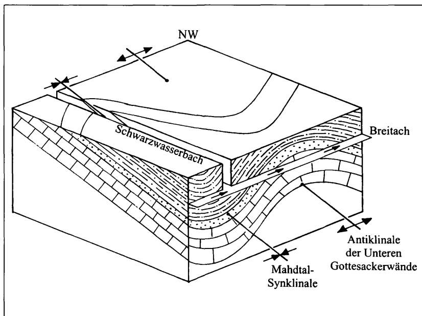
Abb. 13: Schematisches geologisches Blockbild des unteren Schwarzwassertaales und der Breitachschlucht bei Außerschwende: Im Kern der abtauchenden Mahdtal-Synklinale bedecken die wasserstauenden Leistmergel den aus Schrattenkalk bestehenden Karstgrundwasserleiter und bilden daher ein artesisches System. Dort wo die Antiklinale der Unteren Gottesackerwände unter das Breitachtal abtaucht, durchschneidet die Breitach die Leistmergel und den Glaukonitsandstein, so daß auf einer Strecke von ca. 200 m Schrattenkalk ansteht. Dort befindet sich die Grundquelle QG
