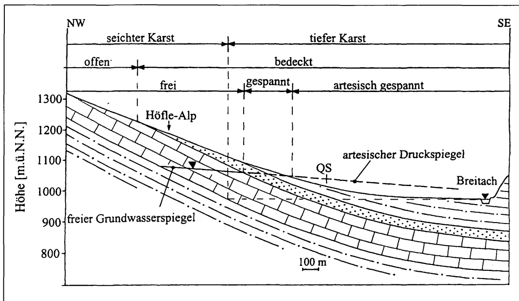
Abb. 6: Schematisches hydrogeologisches Längsprofil durch das Mahdtal und das untere Schwarzwassertal bis zur Breitach, Erläuterung siehe Text
