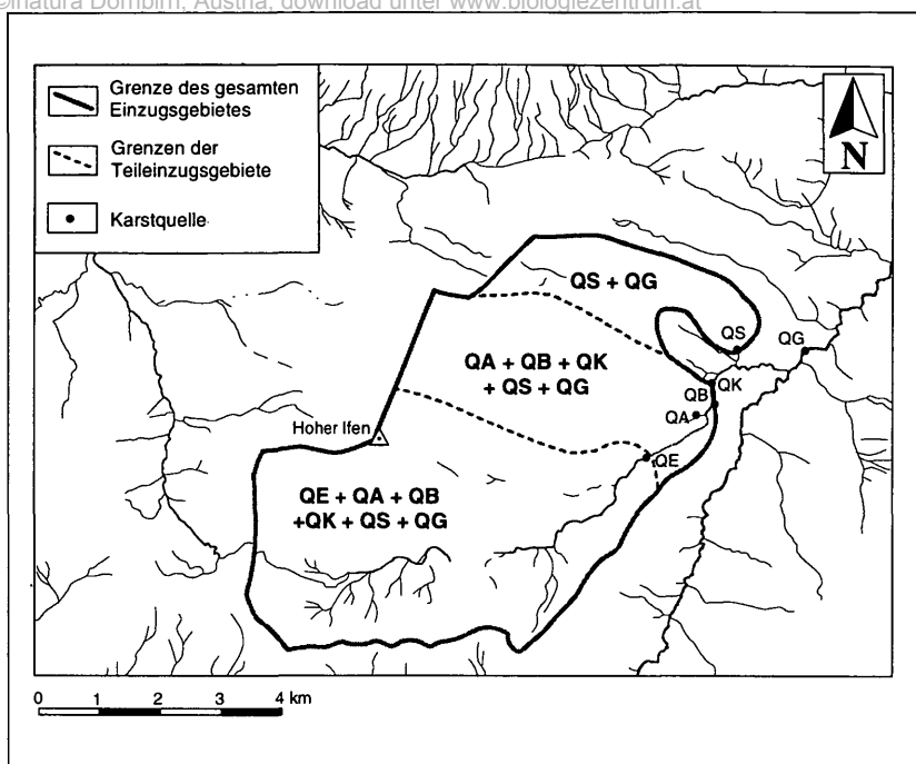
Abb. 24: Einzugsgebiete der Karstquellen: Ein großes, zusammenhängendes Einzugsgebiet wird durch Antiklinalen in Teileinzugsgebiete gegliedert. Bei Niedrigwasser und Versinkung an der Estavelle wird auch die orographisch rechte (südliche) Seite des Schwarzwassertales vollständig von den Karstquellen entwässert
