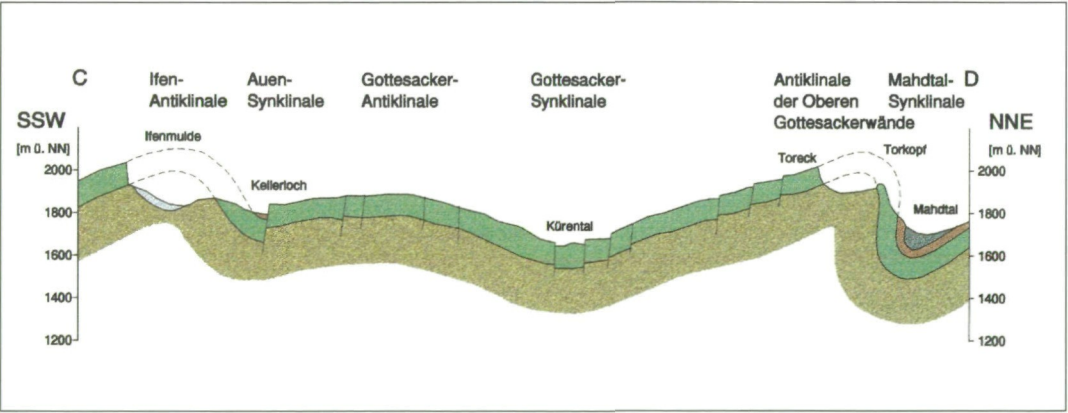
Abb. 3: Geologisches Profil vom Hohen Ifen über den Gottesacker zum Mahdtal. Entlang der Ifen-Antiklinale ist der Schrattekalk aufgebrochen und muldenförmig ausgeräumt, dort befindet sich die Ifenmulde. Auch zwischen Toreck und Torkopf wurde der Schrattekalk abgetragen. Die gesamte Oberfläche des Gottesackers wird von Schrattekalk aufgebaut. Hellbraun: Drusbergsschichten, grün: Schrattekalk, braun: Glaukonitsandstein, oliv: Leistmergel, hellblau: Quartär. Profil erstellt mit ARC/INFO 7.0.4, (GOLDSCHIEDER, 1997)
