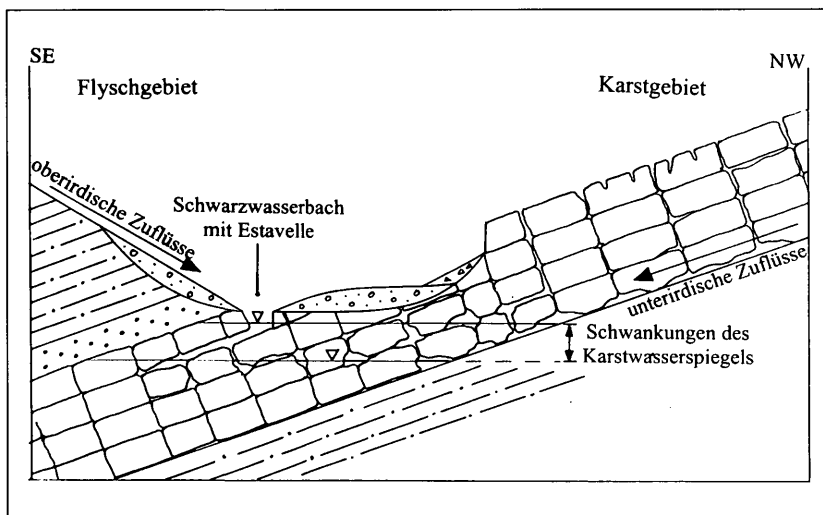
Abb. 23: Schematischer Querschnitt durch das Schwarzwassertal im Bereich der Estavelle. Der Schwarzwasserbach erhält oberirdische Zuflüsse aus dem Flyschgebiet, der Talgrundwasserleiter wird von unterirdischen Zuflüssen aus dem Karst gespeist. Die Estavelle stellt die Verbindung zwischen dem Schwarzwasserbach und dem Grundwasserleiter dar
