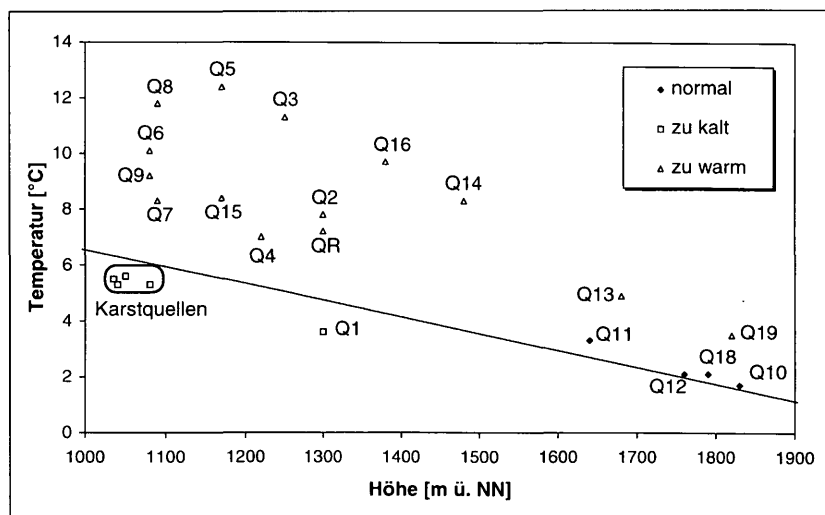
Abb. 15: Durchschnittliche Temperaturen der untersuchten Quellen in Abhängigkeit von der Höhenlage. Die Gerade zeigt den Verlauf der Lufttemperaturen, der aus der Jahresmitteltemperatur der Klimastation Hirschegg ( 5,7^{\circ}\text{C} ) und einer Temperaturabnahme von 0,6^{\circ}\text{C} / 100\text{ m} berechnet wurde. Fast alle Quellen sind deutlich wärmer, als es der jeweiligen Höhenlage entsprechen würde. Die Karstquellen sind zu kalt, da sie Zuflüsse aus einem hochgelegenen Einzugsgebiet erhalten. Lediglich die Quellen Q10, Q11, Q12 und Q18 zeigen der Höhenlage entsprechende Temperaturen
