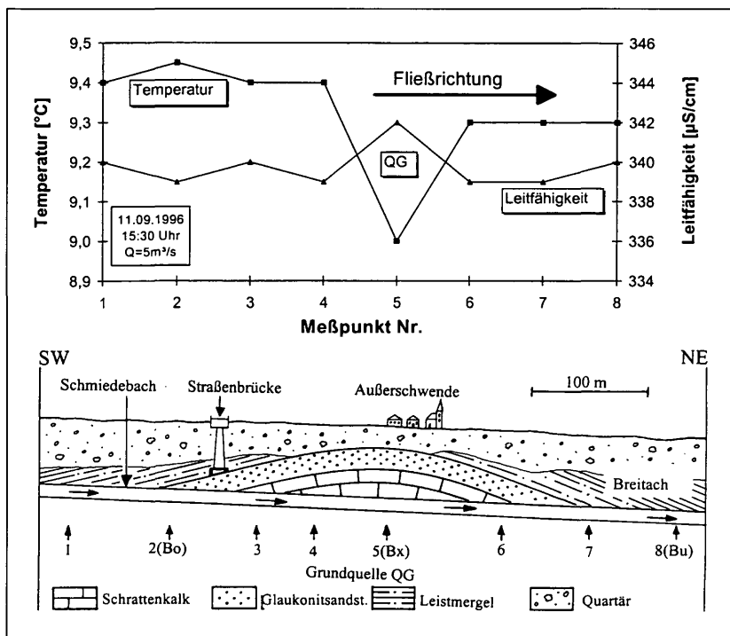
Abb. 14: Geologisches Profil und Profil der Temperatur und Leitfähigkeit im Bereich der vermuteten Grundquelle in der Breitach vom 11.09.1996. Bei P5, also genau im Kern der Antiklinalen ist die Wassertemperatur deutlich erniedrigt, die elektrische Leitfähigkeit ist leicht erhöht. Zwischen P4 und P5 muß sich also die Grundquelle QG befinden
