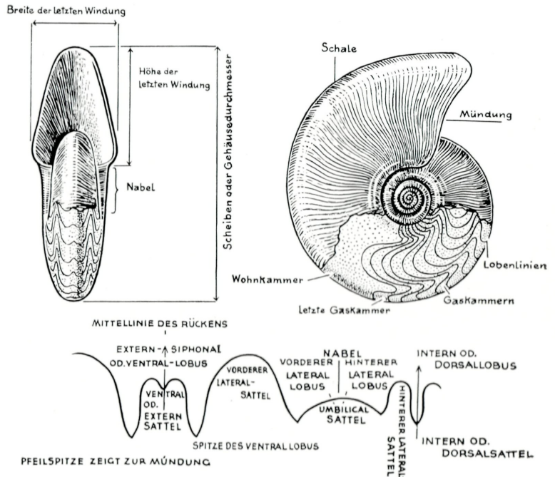
Abb. 6. Das Ammonitengehäuse (nach R. C. Moore)
