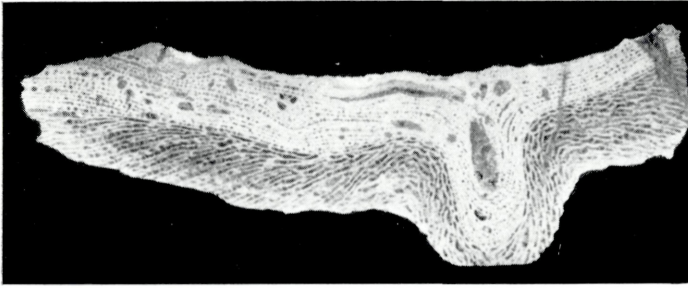
Abb. 4. Stromatoporen überwachsen und töten Bödenkorallen ( Stromatoporella auf Alveolites ). Deutlich sind die in die Höhlungen des Korallenstockes eingedrungenen Hydrozoen zu erkennen. Vertikalschliff. Mitteldevon von Gerolstein in der Eifel (4fache Vergrößerung)
