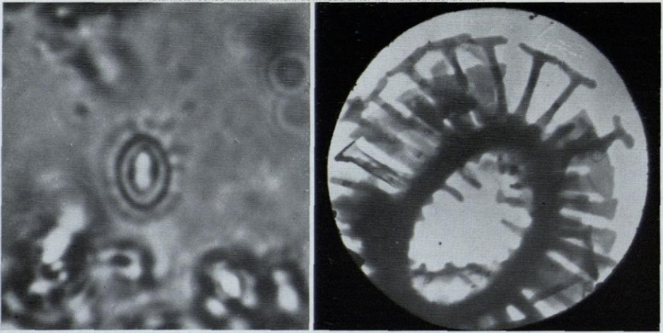
Abb. 28. Pflanzliche Mikroorganismen — Kalkflagellaten ( Coccolithus huxleyi [Lohm.] Kpt.). Links: Coccolith in Flächenansicht in 5400facher Vergrößerung, aus dem Bodenschlamm des Golfs von Neapel. Rechts: Coccolith der gleichen Spezies. Aufnahme im Elektronenmikroskop, in 24.600facher elektronenoptischer Vergrößerung. Globigerinenschlamm der Station 172 der „Valdivia“-Expedition (Indischer Ozean)
