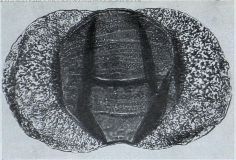
Abb. 32. Mikrospore eines Farnsamers? ( Lueckisporites richteri Klaus) aus dem alpinen Salzgebirge von Hallstatt (Ober-Perm), 660fach vergrößert. Es sind die Einzelheiten der Luftsäcke und des Zentralkörpers zu sehen (Inkohlte Membran) Aufnahme Prof. Dr. W. Klaus
