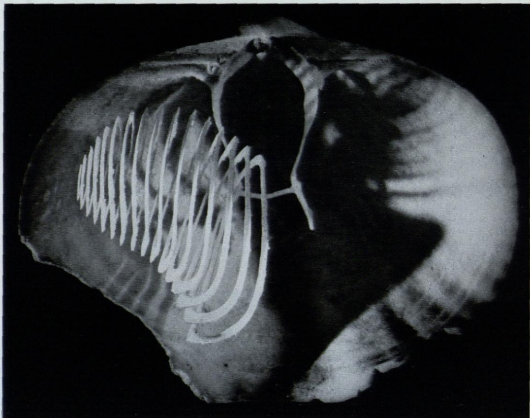
Abb. 35. Ein Beispiel für ausgezeichnete fossile Erhaltung. Bei diesem Brachiopoden ( Spiriferina pinguis Ziet.) ist auf der linken Seite noch das zarte Armgerüst erhalten. Die Spiralkegel sind bei den Brachiopoden mittels Leisten (Cruren) an der Schale befestigt. Das Exemplar stammt aus dem unteren Jura (mittleren Lias) von Frankreich. Die Schale ist 35 mm breit
