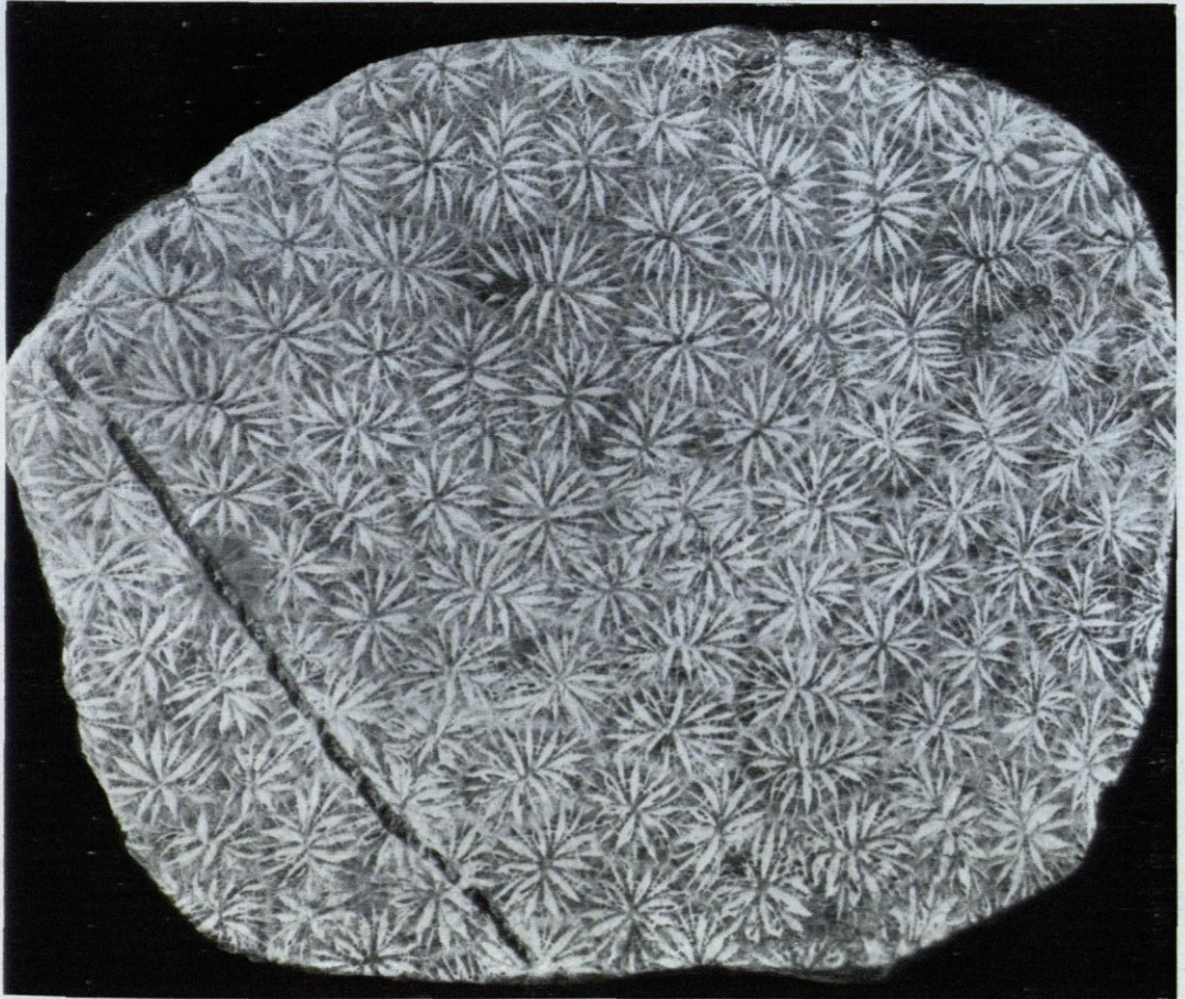
Abb. 34. Querschnitt (Anschliff) eines Korallenstockes von Palaeastraea grandissima (Frech) aus der oberen Trias (Zlambach-Schichten) von Alt-Aussee in Steiermark (annähernd natürliche Größe)
