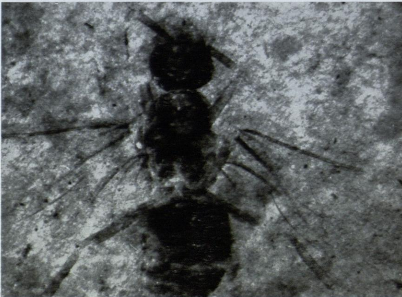
Abb. 39. Ameisenrest ( Myrmecinae -Art) aus den Süßwasserablagerungen (Jungtertiär) von Weingraben bei Draßmarkt im Burgenland. In diesen bentonitischen Tonen sind sogar die zarten Flügel ausgezeichnet erhalten. Ungefähr 8fach vergrößert. (Gesammelt von Peter Ullrich).
