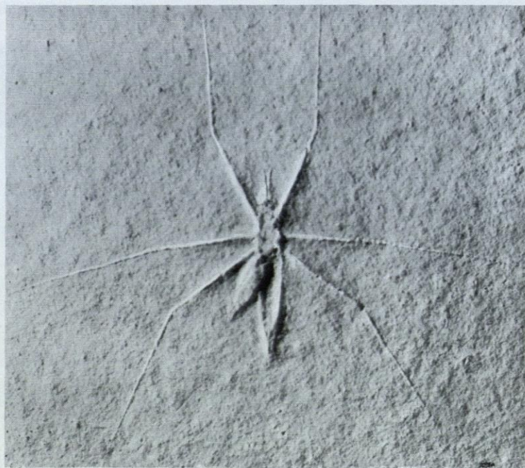
Abb. 37. Abdruck eines Geradflüglers (Orthoptera) im „Lithographischen Schiefer“ (Ober-Malm) von Eichstätt, Bayern. Chresmoda obscura Germar. Dieses Insekt ist vielleicht ein Vorläufer der Fangheuschrecken (Mantiden) und der Gespensterheuschrecken (Phasmiden) (verkleinert)
