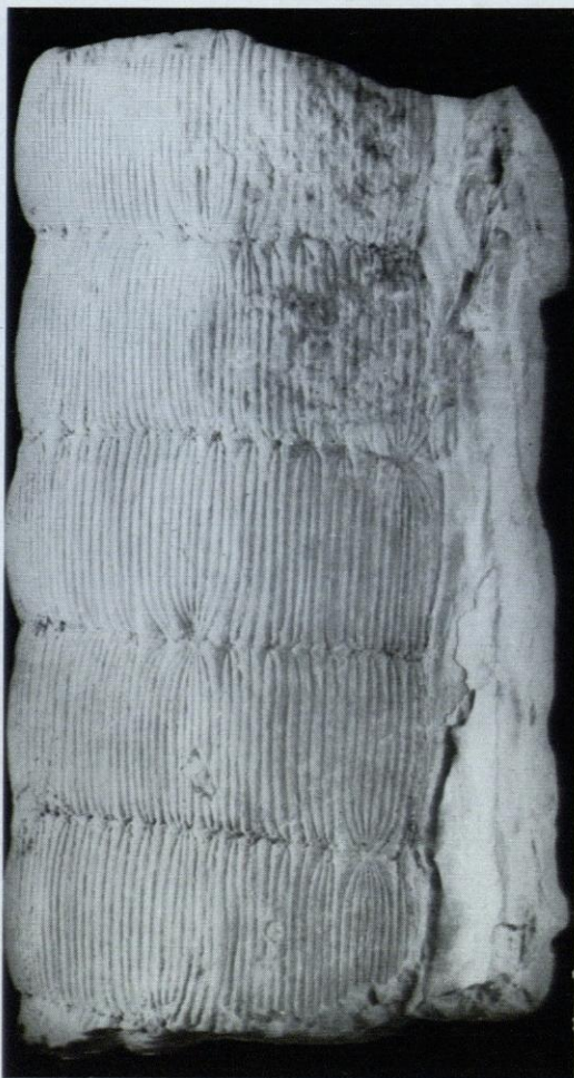
Abb. 31. Steinkern (Ausfüllung eines Markhohlraumes) des Stammes eines Schachtelhalmgewächses, Calamites (Eucalamites) cruciatus Brongn., aus dem Ober-Karbon von Saarbrücken (stark verkleinert)
