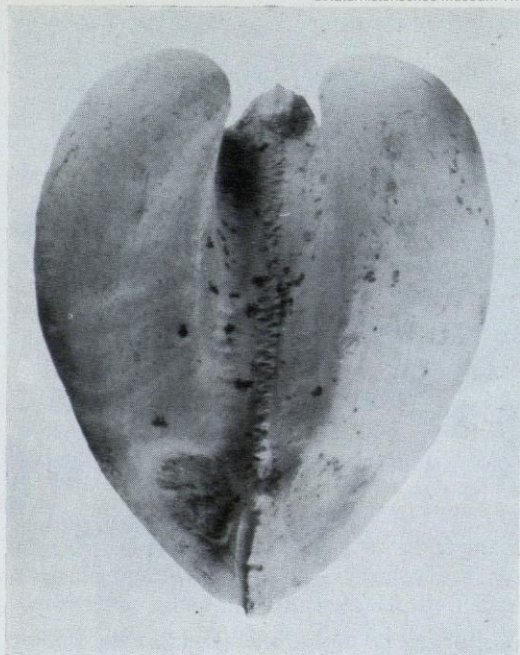
Abb. 36. Steinkern einer Muschel ( Isoarca explicata longa Boehm). Ansicht von oben. Es sind sowohl die Muskeleindrücke als auch die Zähne des Schloßapparates abgeformt und deutlich zu sehen. Das Exemplar stammt aus dem Kalkstein (Ober-Malm) von Ernstbrunn in Niederösterreich (natürliche Größe)
