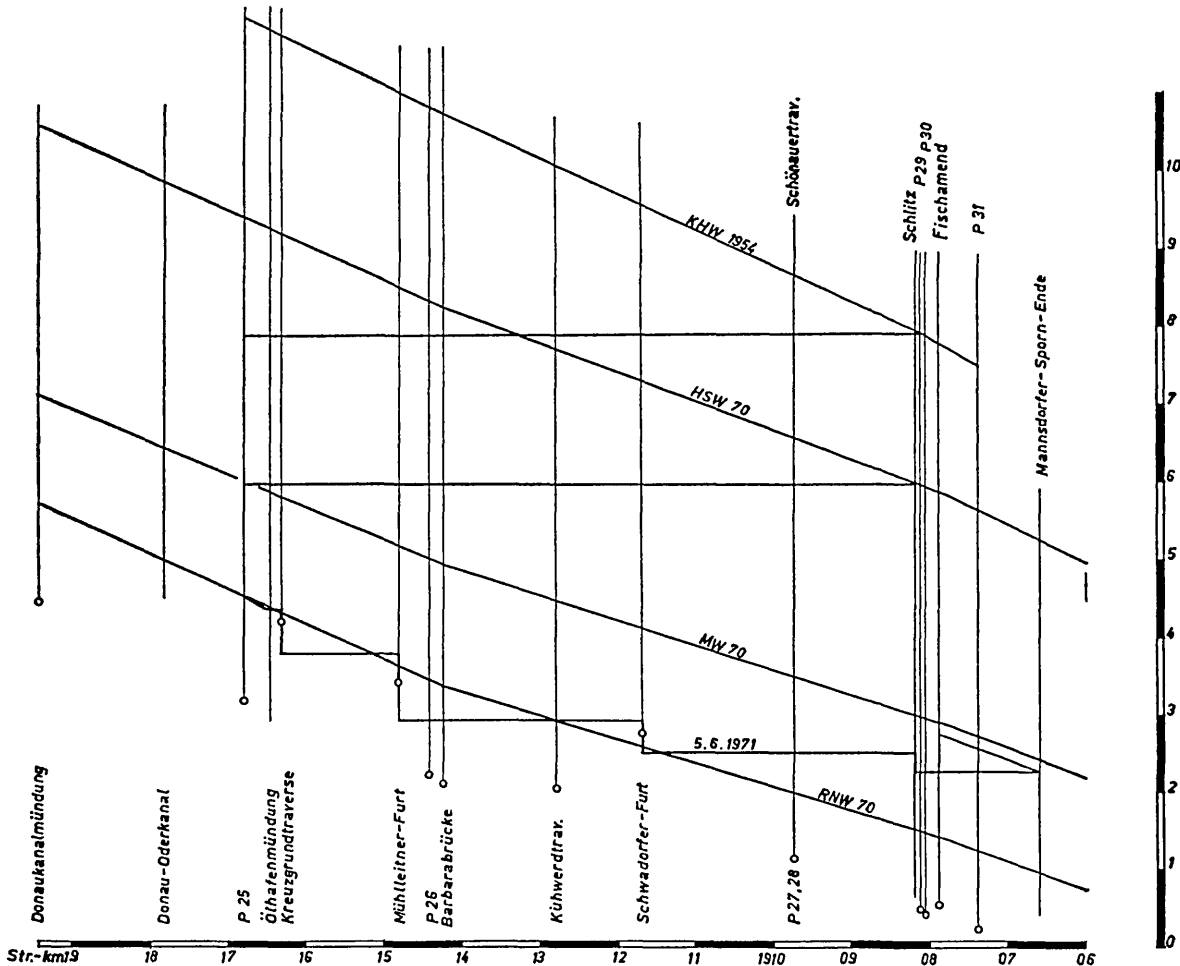
Abb. 2: Die hydrologischen Verhältnisse bei kennzeichnenden Wasserständen der Donau im Rückstaugebiet Mülhleitner-Schnöau
