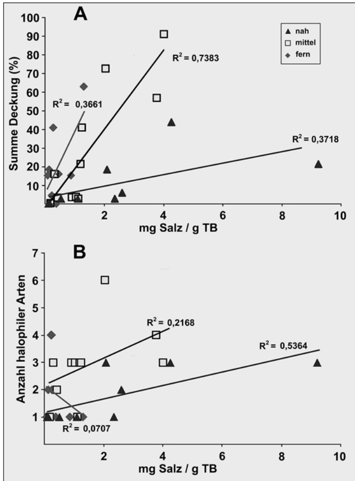
Abb. 19: Halophile Arten (mit ELLENBERG'schen Salz-Zeigerwerten über 5) in den drei unterschiedlich vom Stall entfernten Zonen der Hutweide in Abhängigkeit vom Bodensalzgehalt. A Gesamtdeckung, B Anzahl der Arten, mit Trendlinie und Bestimmtheitsmaß R^2 ; jedes Symbol entspricht einer Aufnahme. – Fig. 19: Halophytic plant species (with salt pointer values above 5 following ELLENBERG) within the three zones in different distances to the stable depending on the soil salt content. A. total covering, B. number of species with trend line and stability index; each symbol corresponds to one single phytosociological recording.
