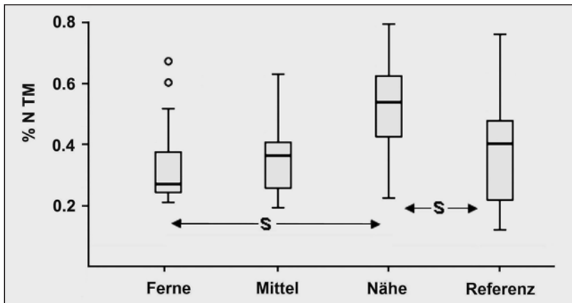
Abb. 6: Gesamt-N-Gehalte in Böden der Hutweide Lange Lacke (Erklärung siehe Abb. 3). – Fig. 6: Total Nitrogen contents in soils of the „Hutweide Lange Lacke“ (for explanations see fig. 3).
