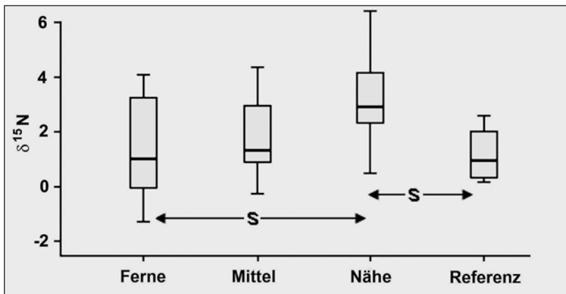
Abb. 7: \delta^{15}N -Werte in Böden der Hutweide Lange Lacke (Erklärung siehe Abb. 3). – Fig. 7: \delta^{15}N -values in soils of the „Hutweide Lange Lacke“ (for explanations see fig. 3).
