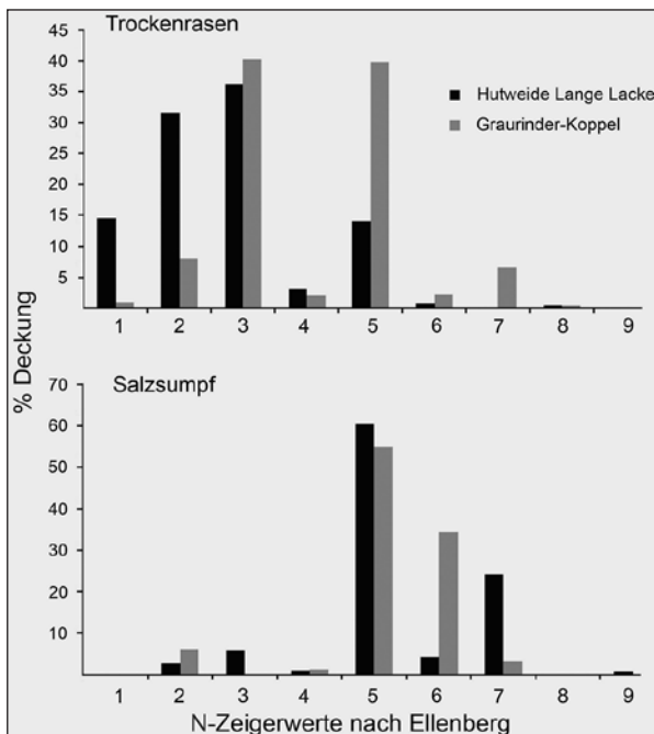
Abb. 16: N-Zeigerwert-Analyse für die Habitate Trockenrasen und Salzsumpf in der Hutweide Lange Lacke und in der Graurinder-Koppel. Die auf die Hutweide bezogenen Balken entsprechen den Mittelwerten der Deckungen auf den Probeflächen aller drei unterschiedlich weit vom Stall entfernten Zonen. – Fig. 16: Application of nitrogen pointer values following ELLENBERG to the habitats „Trockenrasen“ (dry meadow) and „Salzsumpf“ (saline bog) in the „Hutweide Lange Lacke“ and the „Graurinder-Koppel“. The bars corresponding to the „Hutweide“ are mean covering values of species from the plots within all three zones in different distances to the stable (for additional explanations see fig. 9 and chapter Material and Methods).
