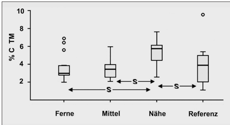
Abb. 8: Gesamtgehalte an organischem Kohlenstoff in Böden der Hutweide Lange Lacke (Erklärungen siehe Abb. 3). – Fig. 8: Total organic carbon contents in soils of the „Hutweide Lange Lacke“ (for explanations see fig. 3).
