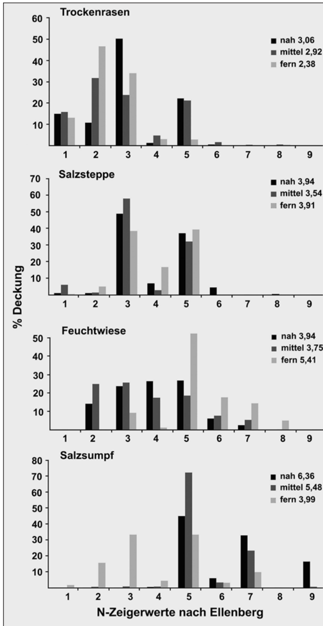
Abb. 9: N-Zeigerwert-Analyse für die vier Habitate in allen 3 Zonen der Hutweide Lange Lacke. Die Balkenhöhe entspricht der Summe der rechnerisch ermittelten durchschnittlichen Deckungswerte aller Arten in einer bestimmten Zone mit dem jeweils gleichen N-ZW. Zusätzlich ist der durchschnittliche N-ZW sämtlicher in einer bestimmten Zone angetroffenen Arten angeführt. – Fig. 9: Application of nitrogen pointer values following ELLENBERG to the four habitats in all 3 zones within the „Hutweide Lange Lacke“. The length of the bars corresponds to the sum of the calculated average cover of species within a distinct zone showing the same nitrogen pointer value. Additionally, the mean N pointer value of all plant species observed in a distinct zone is shown.
