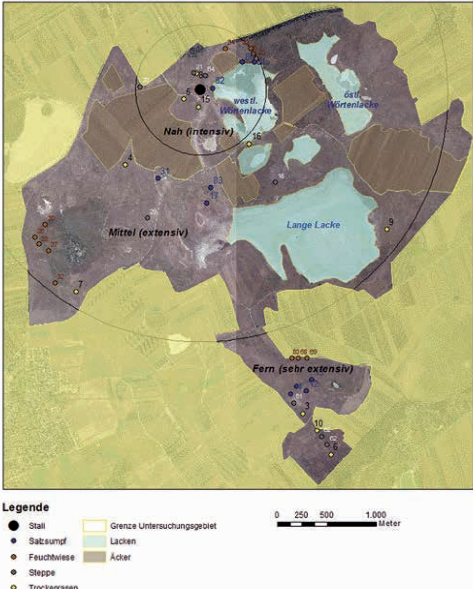
Abb. 1: Aufnahmeflächen in der Hutweide Lange Lacke. Details zu den nummerierten Flächen finden sich in STEINGRUBER (2014). – Fig 1: Plots in the „Hutweide Lange Lacke“. For details concerning the numbers see STEINGRUBER (2014).
