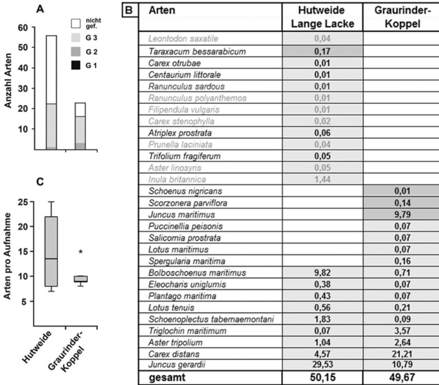
Abb. 18: Verteilung der Pflanzenarten im Habitat Salzsumpf auf der Hutweide Lange Lacke und in der Graurinder-Koppel (Erklärungen siehe Abb. 17). – Distribution of plant species in the habitat „Salzsumpf“ (saline bog) in the „Hutweide Lange Lacke“ and in the „Graurinder-Koppel“ (for explanations see fig. 17).
