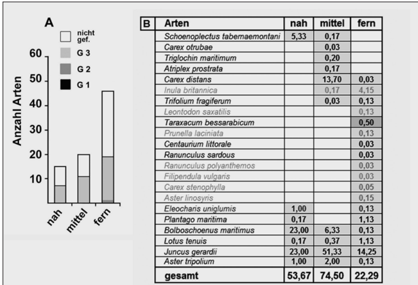
Abb. 13: Verteilung der Pflanzenarten im Habitat Salzsumpf innerhalb der Hutweide Lange Lacke (Erklärung siehe Abb. 10). – Fig. 13: Distribution of plant species in the habitat „ Salzsumpf “ (saline bog) in the „Hutweide Lange Lacke“ (for explanations see fig. 10).
