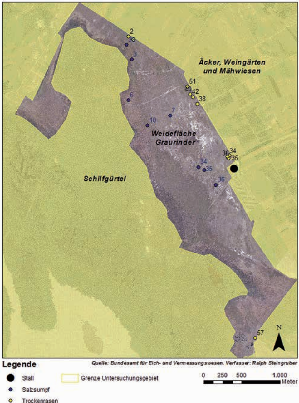
Abb. 2: Aufnahmeflächen in der Graurinder-Koppel. Details zu den nummerierten Flächen finden sich in STEINGRUBER (2014). – Fig. 2: Plots within the paddock of Hungarian cows („Graurinder-Koppel“). For details concerning the numbers see STEINGRUBER (2014).
