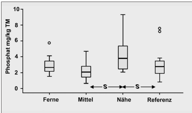
Abb. 3: Phosphat-Gehalte in Böden der Hutweide Lange Lacke. Mittelwerte von Böden aller 4 Habitate (Boxplot-Darstellung mit Median und Standardfehler). Signifikante ( p > 0,05 ) Unterschiede sind mit s, Ausreißer mit o markiert. Die Referenz-Werte beziehen sich auf Böden unbeweideter, aber vergleichbarer Habitate außerhalb der Hutweide. – Fig. 3: Phosphate content in soils of the „Hutweide Lange Lacke“. Mean values of soils of all 4 habitats (boxplots with median and standard error). Significant differences ( p > 0,05 ) are marked with s, outliers with o. Reference values refer to soils of ungrazed plots outside of the “Hutweide”.
