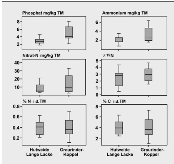
Abb. 14: Vergleich der Boden-Nährstoffe im Habitat Trockenrasen zwischen Hutweide Lange Lacke und Graurinder-Koppel. Boxplot-Darstellung mit Median, Quartilen sowie Minimum- und Maximum-Werten. – Fig 14: Comparison of soil nutrients in the habitat „Trockenrasen“ (dry meadow) between „Hutweide Lange Lacke“ and „Graurinder-Koppel“. Box-plot showing median, quartils, minimum and maximum values.
