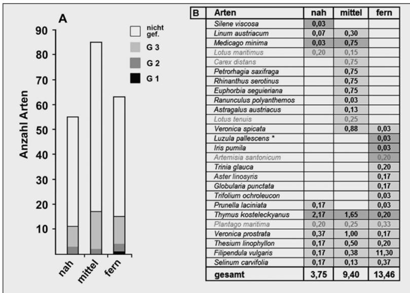
Abb. 10: Verteilung der Pflanzenarten im Habitat Trockenrasen innerhalb der Hutweide Lange Lacke. A. Anzahl Arten nach Gefährdungsstatus: G 1 = in Gefahr des Aussterbens bedroht, G 2 = stark gefährdet, G 3 = gefährdet. B. Gefährdete Arten mit ihren durchschnittlichen Deckungswerten: hellgraue Felder = G 3 – Arten, dunkelgraue Felder = G 1 (mit Sternchen) und G 2-Arten zusammengefasst; graue Artnamen beziehen sich auf Arten, die ihren Schwerpunkt in einem anderen Habitat haben. Erläuterung zu den Deckungswerten siehe Kap. Material und Methodik. – Fig. 10: Distribution of plant species in the habitat „Trockenrasen“ (dry meadow) in the “Hutweide Lange Lacke”. A. Species number according to the endangering status: G 1 = in danger of extinction, G 2 = highly endangered G 3 = endangered. B. Endangered species and their average covering values: weak gray = G 3 – species, dark gray = G 1 (with asterisks) and G 2 species combined; gray labelling of species names correspond to species with preferential distribution in an other habitat. Explanations to the covering values see chapter Material and Methods.
