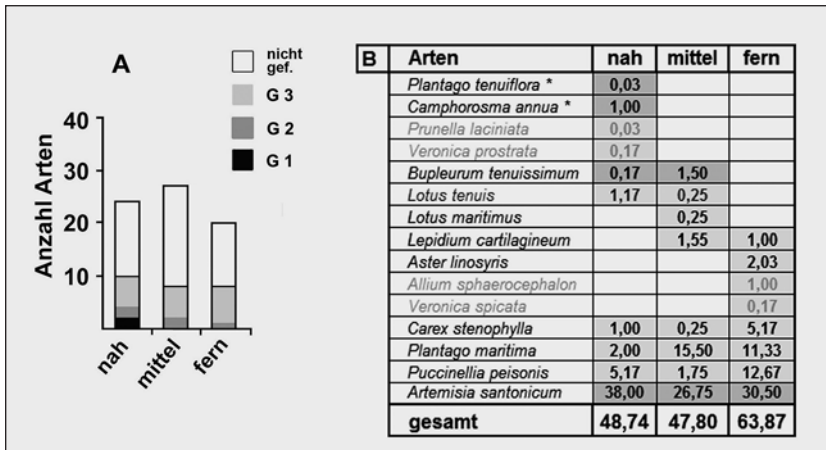
Abb. 11: Verteilung der Pflanzenarten im Habitat Salzsteppe innerhalb der Hutweide Lange Lacke (Erklärung siehe Abb. 10). – Fig. 11: Distribution of plant species in the habitat „Salzsteppe“ (saline steppe) in the „Hutweide Lange Lacke“ (for explanations see fig. 10).
