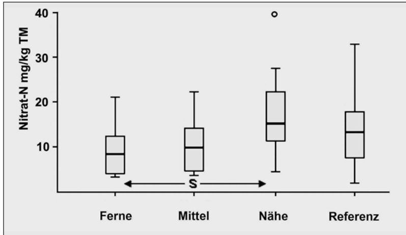
Abb. 4: Nitrat-N-Gehalte in Böden der Hutweide Lange Lacke (Erklärung siehe Abb. 3). – Fig. 4: Nitrate-N-contents of soils in the „Hutweide Lange Lacke“ (for explanations see fig. 3).
