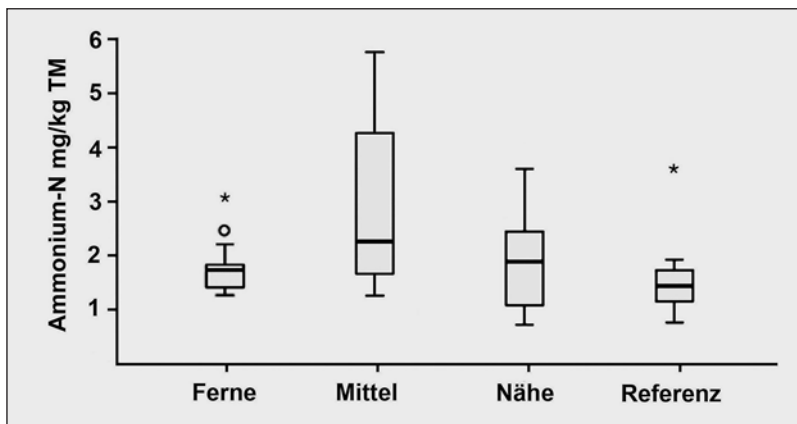
Abb. 5: Ammonium-N-Gehalte in Böden der Hutweide Lange Lacke (Erklärung siehe Abb. 3). – Fig. 5: Ammonium-N-contents in soils of the „Hutweide Lange Lacke“ (for explanations see fig. 3).
