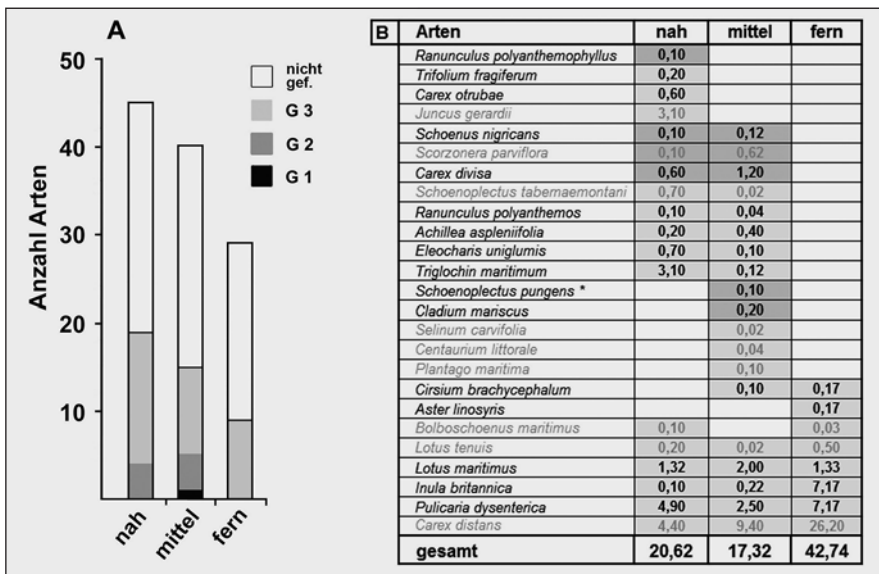
Abb. 12: Verteilung der Pflanzenarten im Habitat Feuchtwiese innerhalb der Hutweide Lange Lacke (Erklärung siehe Abb. 10). – Fig. 12: Distribution of plant species in the habitat „Feuchtwiese“ (wet meadow) in the „Hutweide Lange Lacke“ (for explanations see fig. 10).
