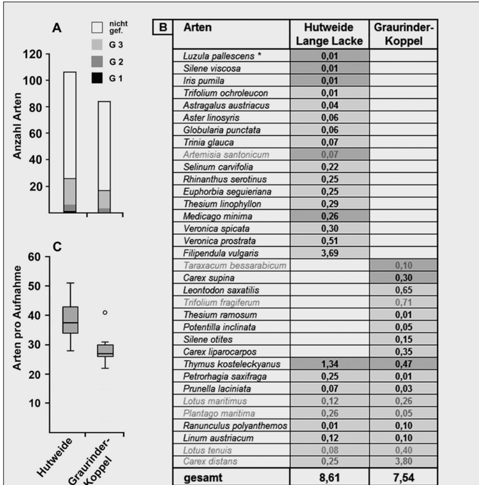
Abb. 17: Verteilung der Pflanzenarten im Habitat Trockenrasen auf der Hutweide Lange Lacke und in der Graurinder-Koppel. A. Anzahl Arten nach Gefährdungsstatus: G 1 = vom Aussterben bedroht, G 2 = stark gefährdet, G 3 = gefährdet. B. Gefährdete Arten mit ihren durchschnittlichen Deckungswerten: hellgraue Felder = G 3 – Arten, dunkelgraue Felder = G 1 (mit Sternchen) und G 2-Arten zusammengefasst; graue Artnamen beziehen sich auf Arten, die ihren Schwerpunkt in einem anderen Habitat haben. C. Artenzahlen pro Aufnahme. Im Fall der Hutweide wurden alle drei Zonen in unterschiedlicher Stallentfernung gemeinsam verrechnet. Erläuterung zu den Deckungswerten siehe Kap. Material und Methodik. – Fig. 17: Distribution of plant species in the habitat „ Trockenrasen “ (dry meadow) in the “Hutweide Lange Lacke”. A. Species number according to the endangering status: G 1 = in danger of extinction, G 2 = highly endangered G 3 = endangered. B. Endangered species and their average covering values: weak gray = G 3 – species, dark gray = G 1 (with asterisks) and G 2 species combined; gray labelling of species names corresponds to species with preferential distribution in an other habitat. C. Number of species per phytosociological recording. The plant species from all three zones of the “Hutweide” in different distances to the stable were included. Regarding the covering values see chapter Material and Methods.
