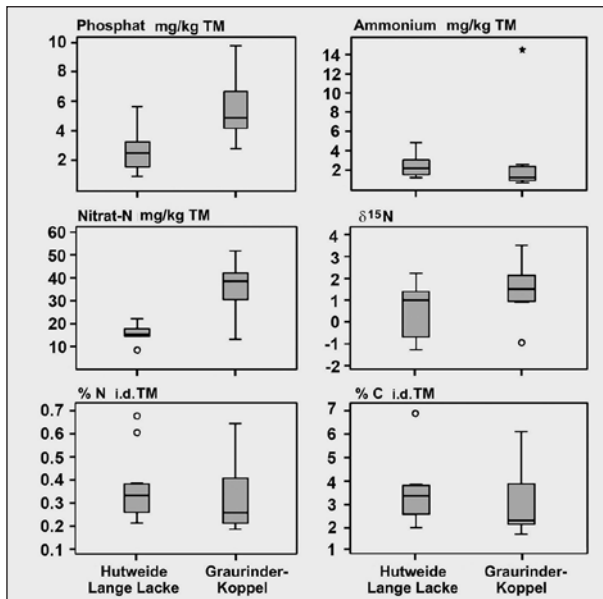
Abb. 15: Vergleich der Boden-Nährstoffe im Habitat Salzsumpf zwischen Hutweide Lange Lacke und Graurinder-Koppel. Erklärung siehe Abb. 14. – Fig 15: Comparison of soil nutrients in the habitat „Salzsumpf“ (saline bog) between „Hutweide Lange Lacke“ and „Graurinder-Koppel“. For explanations see Fig. 14.
