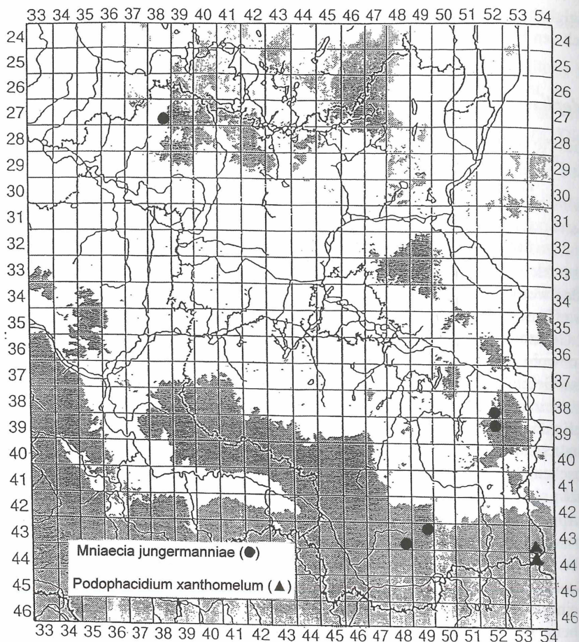
Abb. 1: Bisher bekannte Fundorte von Mniaecia jungermanniae und Podophacidium xanthomelum in Brandenburg.
