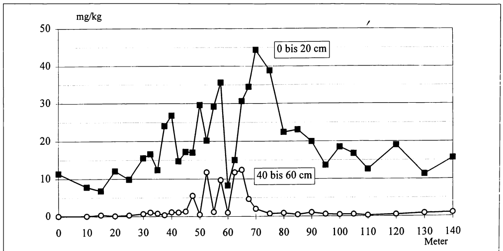
Abb. 1 Cadmiumkonzentrationen in zwei Tiefenstufen entlang eines Transektes.
