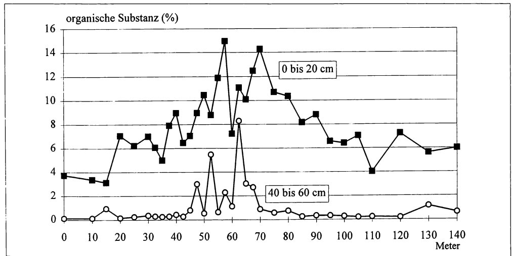
Abb. 2 Gehalte an organischer Substanz in zwei Tiefenstufen entlang eines Transektes.
