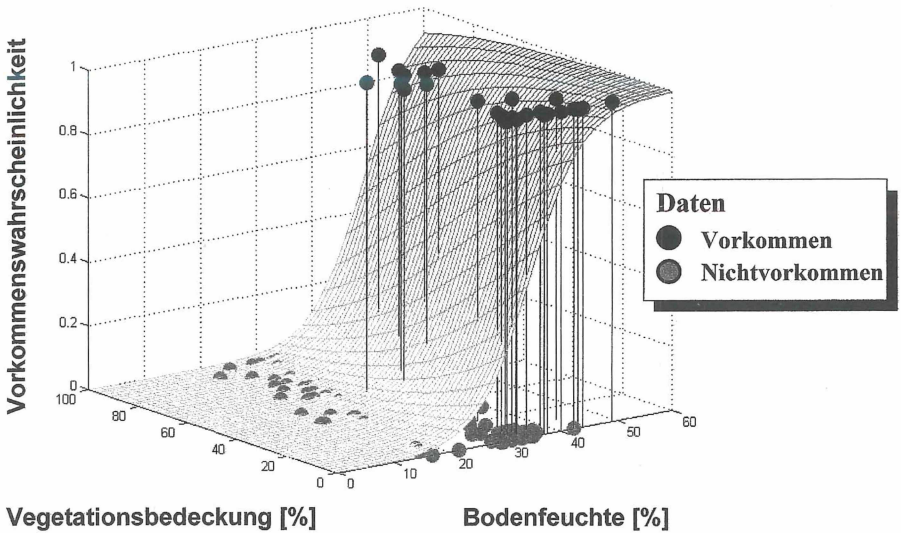
Abb. 2: Responseoberfläche der Vorkommenswahrscheinlichkeit von Agonum livens in Abhängigkeit von Bodenfeuchte und Vegetationsbedeckung. Dargestellt sind auch die zugehörigen Präsenz-Absenz-Daten.
