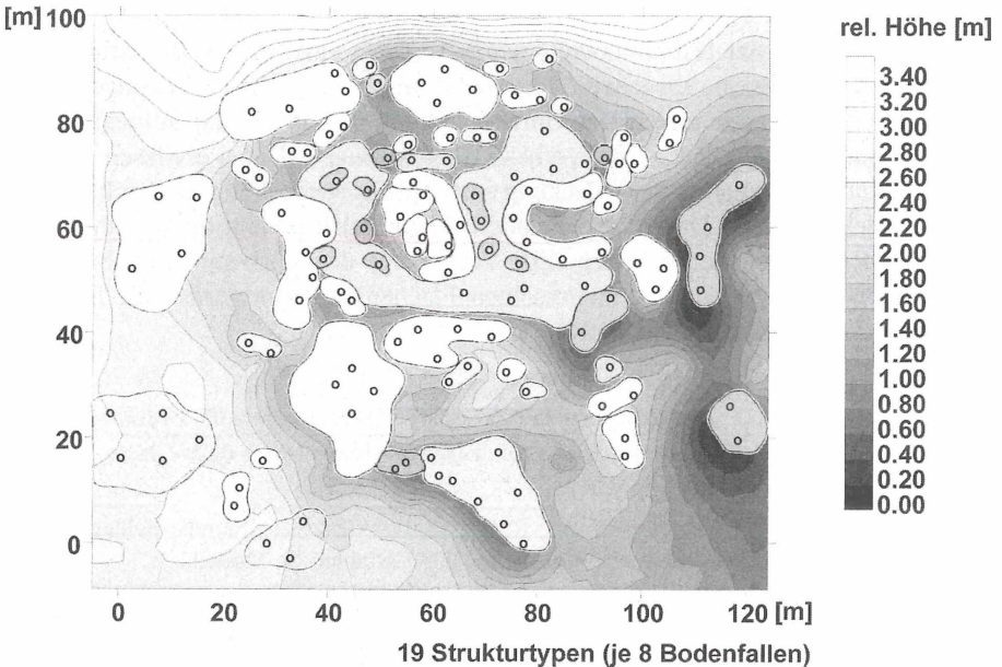
Abb. 1: Skizze des stratifizierten Versuchsdesigns in einer Auwaldparzelle von 100 \times 120 \text{ m}^2 . Das strukturreiche Relief wird durch Höhenlinien mit einer Spanne von 3,40 m gekennzeichnet. Feuchte Senken mit temporären Qualmwassertümpeln und Seggenriedern sind moosartig mit erhöhten, trockeneren Bereichen mit Laubwaldvegetation verzahnt. Je acht Bodenfallen (markiert durch o, \Sigma 152) wurden in 19 zuvor kartierten Vegetationsstrukturtypen (verschiedene Graustufen) über 28 Tage plaziert.
