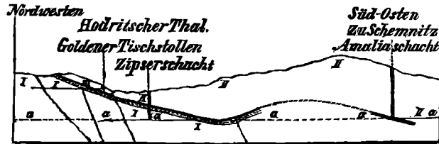
a) Kaiser Josephi II di Erbstollen; I. Syenit, II. Grünsteintrachyt, III. Dacit. ———— Aplit und Quarzit; ———— Werfener Schichten ———— Grünsteintrachyt- (Dacit)-Gänge.
