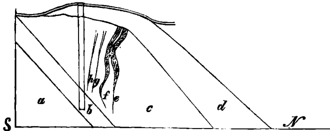
a. Chlorit Thonschiefer. b. Talkschiefer. Quarzit. d. Graphitischer Thonschiefer. e. f. g. h. Bleiglanzgänge.
