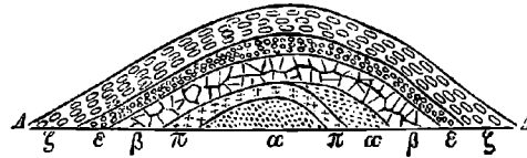
A A Wasserlauf der Sirinnia. α Unterer Lias-Sandstein. β Dunkelgrauer Kalk des Lias. ε Rother Knottenkalk des Tithon. ζ Heller Kalk des Tithon. π Porphyr.
