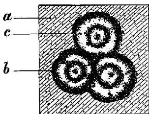
Graphitconcretionen \frac{1}{2} u. G.
