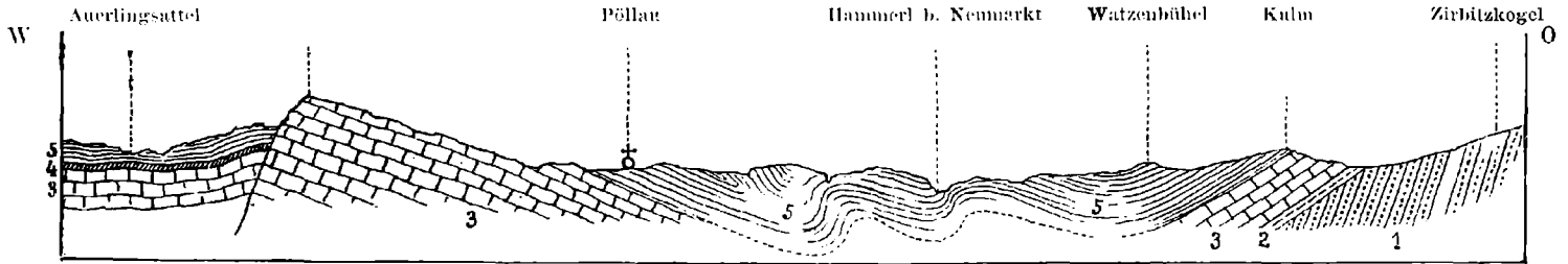
II. Profil durch die Grebenze und die Phyllitmulde von Neumarkt (W-O).
