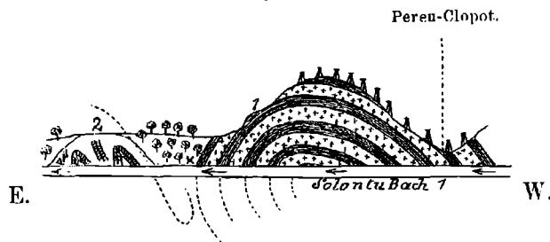
Querprofil des Petroleumfeldes von Solonţu.
