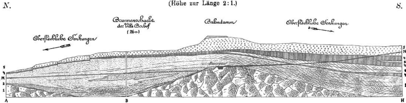
Fig. 1. Stollenprofil durch den Kremserberg: 458 m.
