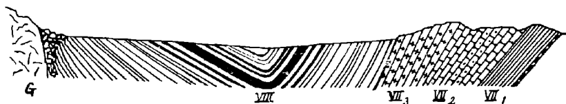
Schematisches Profil durch die Gegend von Djpaló.
