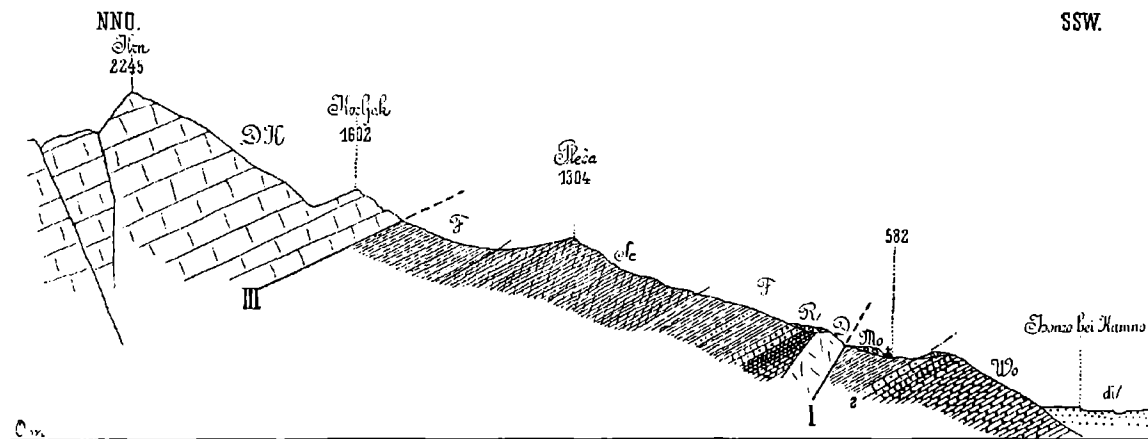
Fig. 4. Profil vom Krn über die Pleča zum Isonzotal bei Kamno.
