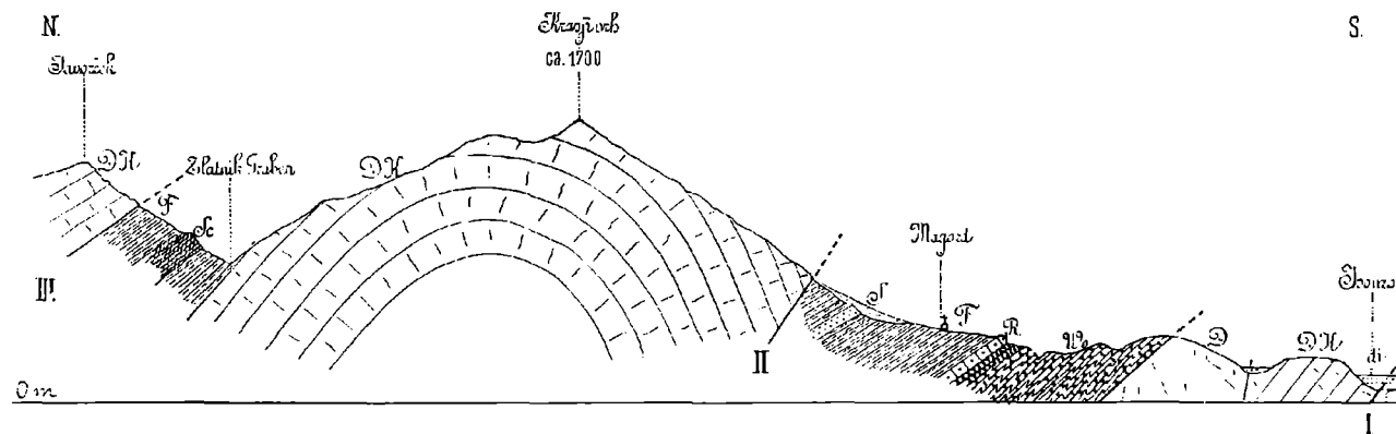
Fig. 3. Profil durch den Krasji vrh (Polovnikgewölbe) zum Isonzo bei Karfreit.
