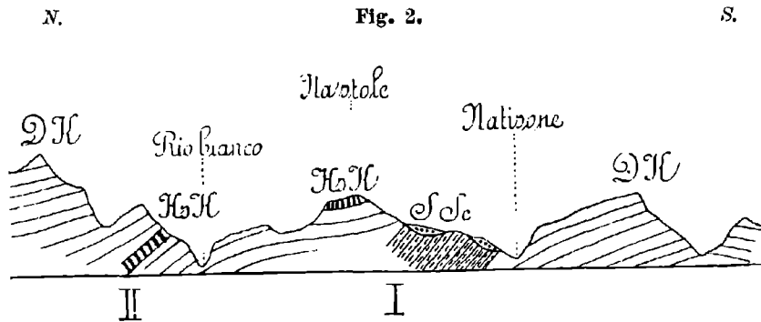
S—N Profil vom Nalonedurchbruch zum Canin. Kopie nach D. Stur, 1858.
