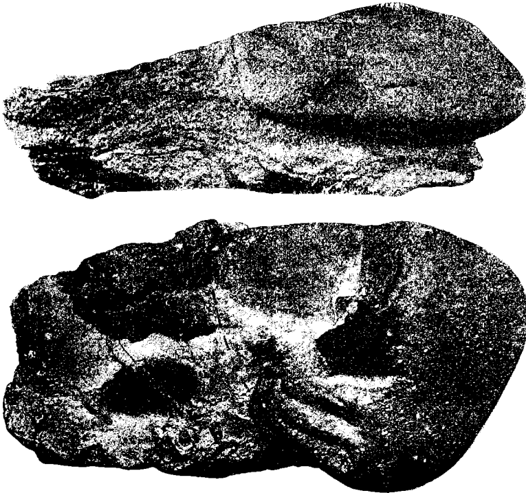
Geröll von Cannelkohle im Karbonsandstein. Natürliche Größe.
