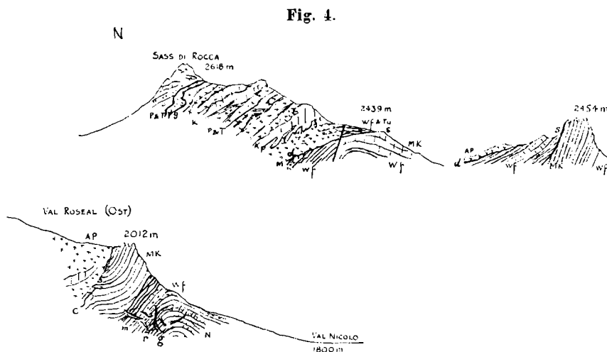
Oben (a) Profil durch den Sasso di Rocca (Südhang). — Maßstab: 1:16.000. Unten (b) Profil unmittelbar östlich von Val Roseal (Südhang des Buffaure).
