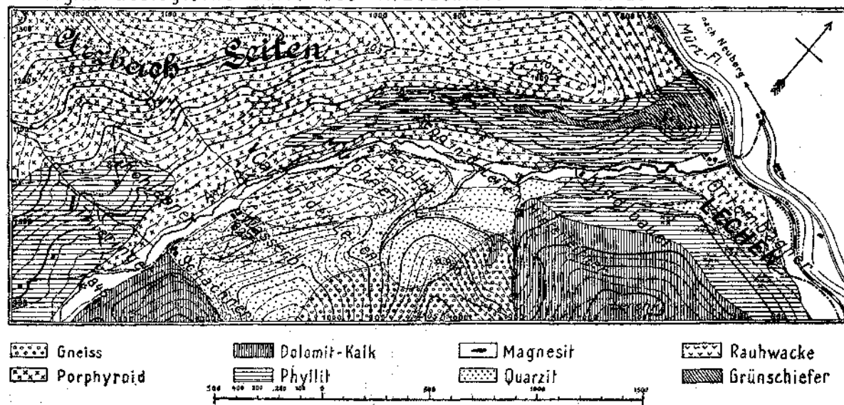
Fig. 2. Geologische Karte des Arzbachtales. Maßstab 1:25.000.
