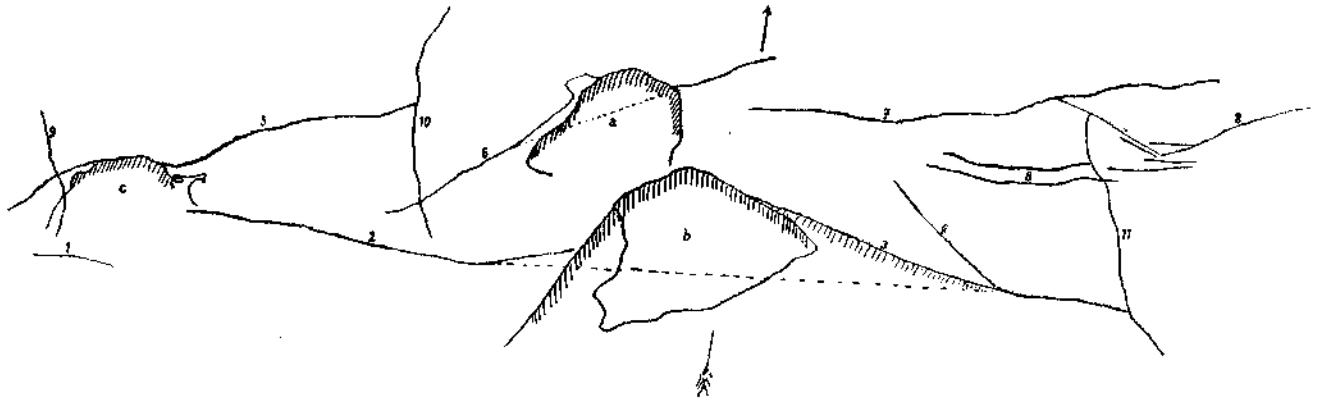
Fig. 1. Oetztaler Phase.
