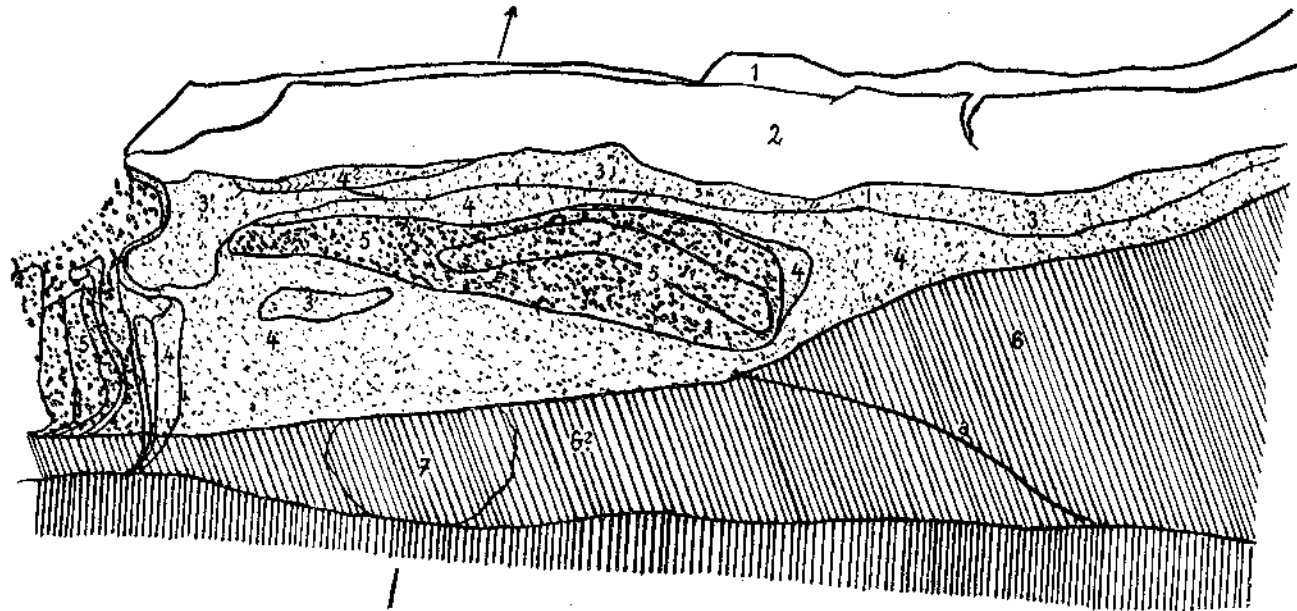
Fig. 2. Tauernphase 1: 3,500.000.
