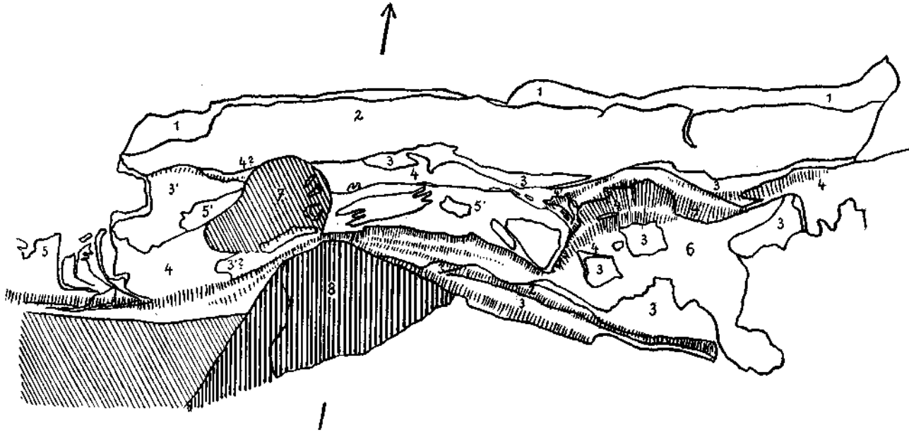
Fig. 3. Jungphase 1 : 3,500.000.
