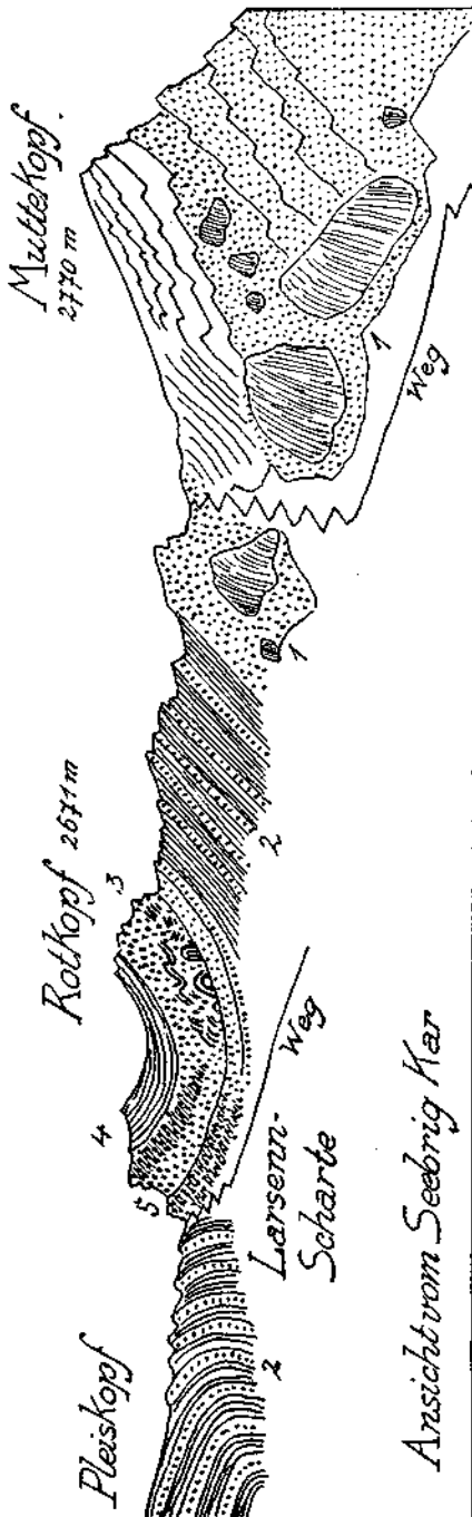
Fig. 7. 1 = Grobe Breccien der Gosauschichten mit reichem evolischem Material und eingebetteten Riesenkalkblöcken. 2 = Massive Breccien, Sandsteine und Mergel, vielfach wechselnd. 3 = Grobe, mächtige Breccien- und Blockschichten mit eingebetteten größeren Faltenstücken. 4 = Massive Breccien. 5 = Rot zementierte Breccien.
