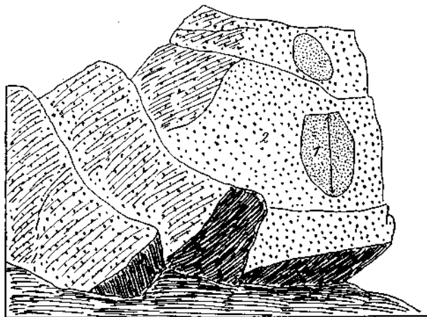
Fig. 5. Gosaublöcke beim Seebrigwasserfall. Einschlüsse von Blöcken einer älteren, feineren Breccie in einer jüngeren, gröberen. Der größere eingeschlossene Block hat einen längeren Durchmesser von zirka 1 m. 1 = Dunkler gefärbte, feinkörnige Breccie mit kleinen roten, grünen, schwarzen Hornsteinstückchen und relativ wenig Kalkzement. 2 = Größere, hellgraue Breccie mit exotischen Geröllen und reichlichem Kalkzement.
