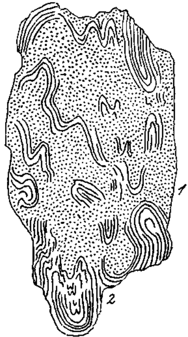
Fig. 8. Beispiel von Ohrmuschelfaltung. Gosablock oberhalb von der Muttekopfhütte. Höhe = \frac{1}{2} m. 1 = Feinere Sand- und Breccienmasse. 2 = Feine kalkige Mergel mit feinsandigen gelblichen Zwischenlagen.
