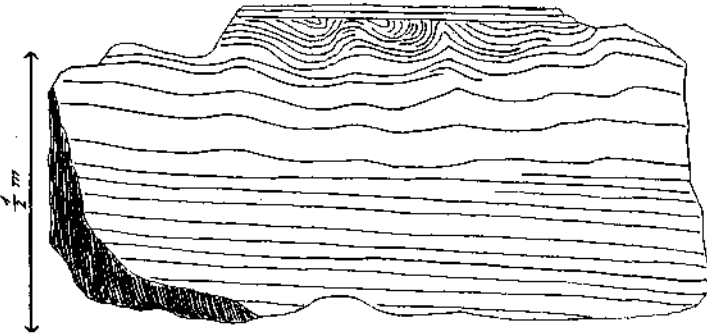
Fig. 9. Gosaublock am Nordhang des Alpjoches. Dunkler, kalkiger Sandstein mit bräunlicher Verwitterung.
