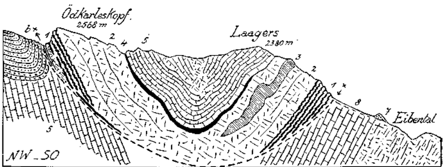
Fig. 2. 1 = Knollen- und Hornsteinkauerkalke, Muschelkalk. 2 =LICHTER Wettersteinkalk. 3 = Rostiger Wettersteindolomit. 4 = Schwarze Schiefer, Sandsteine, Oolithe, dunkle Kalke, Raibler Schichten. 5 = Hauptdolomit, geschichtet und ungeschichtet. 6 = Breccien, Sandsteine, Mergel der Gosauschichten. 7 = Längsmoränenwall aus eckigem Dolomitschutt. 8 = Hangschutt. x-x = Ausstrich der Schubfläche der Krabachjochdecke, welche vorgosauisch gebildet wurde und nachgosauisch eine Belebung erfuhr. Die Krabachjochdecke stellt eine Reliefabschiebung in der Form einer „Mulde ohne Sohle“ vor.
