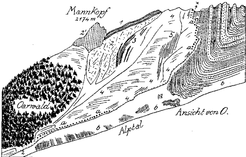
Fig. 1. 1 = Hornsteinkauerkalk, Muschelkalk. 2 = Geschichteter lichter Wettersteinkalk. 2' = Ungeschichteter lichter Wettersteinkalk. 3 = Schwarze Schiefer, Sandsteine, gelblicher Dolomit, Raibler Schichten. 4 = Hauptdolomit. 5 = Schwarzer, dünnplattiger, bituminöser Dolomit. 6 = Breccien, Sandsteine, Mergel der Gosauschichten. a-a = Stellen, wo der Hauptdolomit schön gerundete Dolomitgerölle umschließt. x = Schubfläche der Krabachjochdecke.
