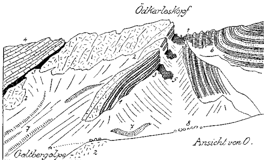
Fig. 3. 1 = Muschelkalk. 2 = Wettersteinkalk. 3 = Raibler Schichten. 4 = Geschichteter Hauptdolomit. 5 = Zertrümmerter Hauptdolomit. 6 = Gosauschichten. 7 = Endmoränen. 8 = Gosaublöcke.
