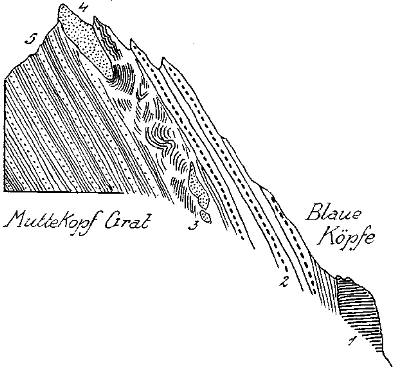
Fig. 6. 1 = Riesenblock aus Oberrätalkalk. 2 = Grobe Breccien mit exotischem Material. 3 = Feine Mergel- und Sandsteinlagen. 4 = Größere Breccienmassen. 5 = Vielfache Wechsellagerung von bunten Breccien mit Mergeln und Sandsteinen.
