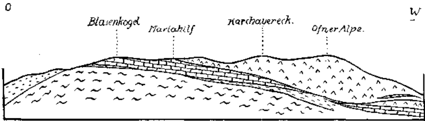
Schematischer O—W Schnitt. Zeichnen siehe Profiltafel.
