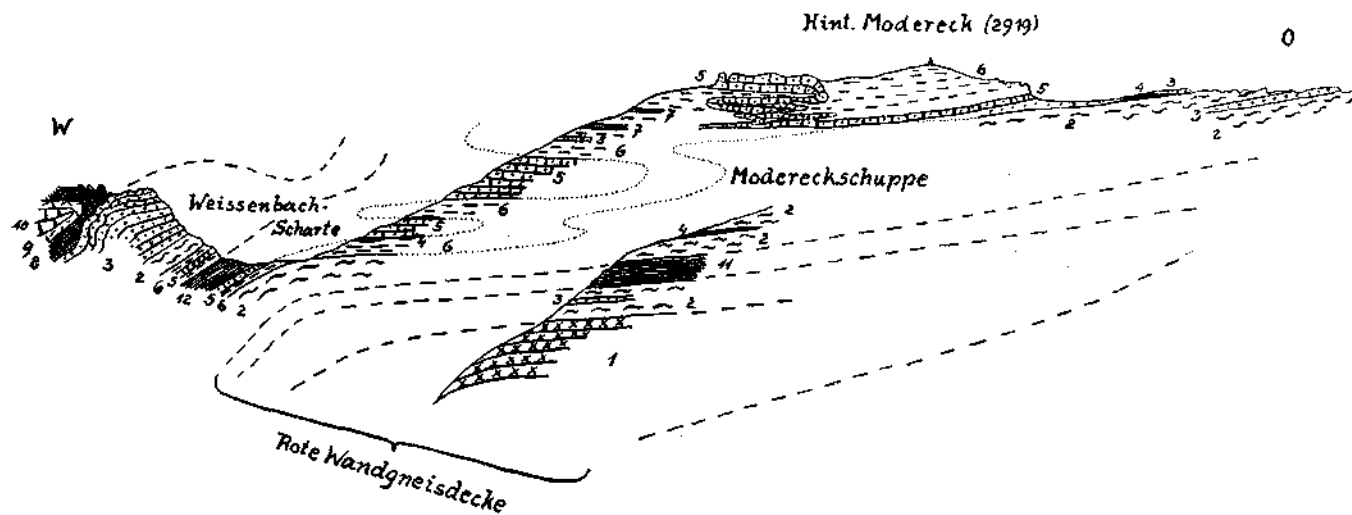
Abb. 1. W—O-Profil über das Hintere Modereck und durch die Karstufe südlich davon. (Etwas vereinfacht.)
