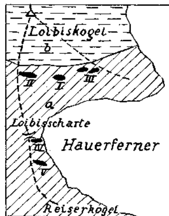
Fig. 1. a = Zone der Eklogite und Eklogitamphibolite. b = Biotitgneise.
