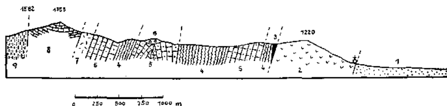
Geologisches Profil: Maria Elend i. R. — Golica-Hütte.
